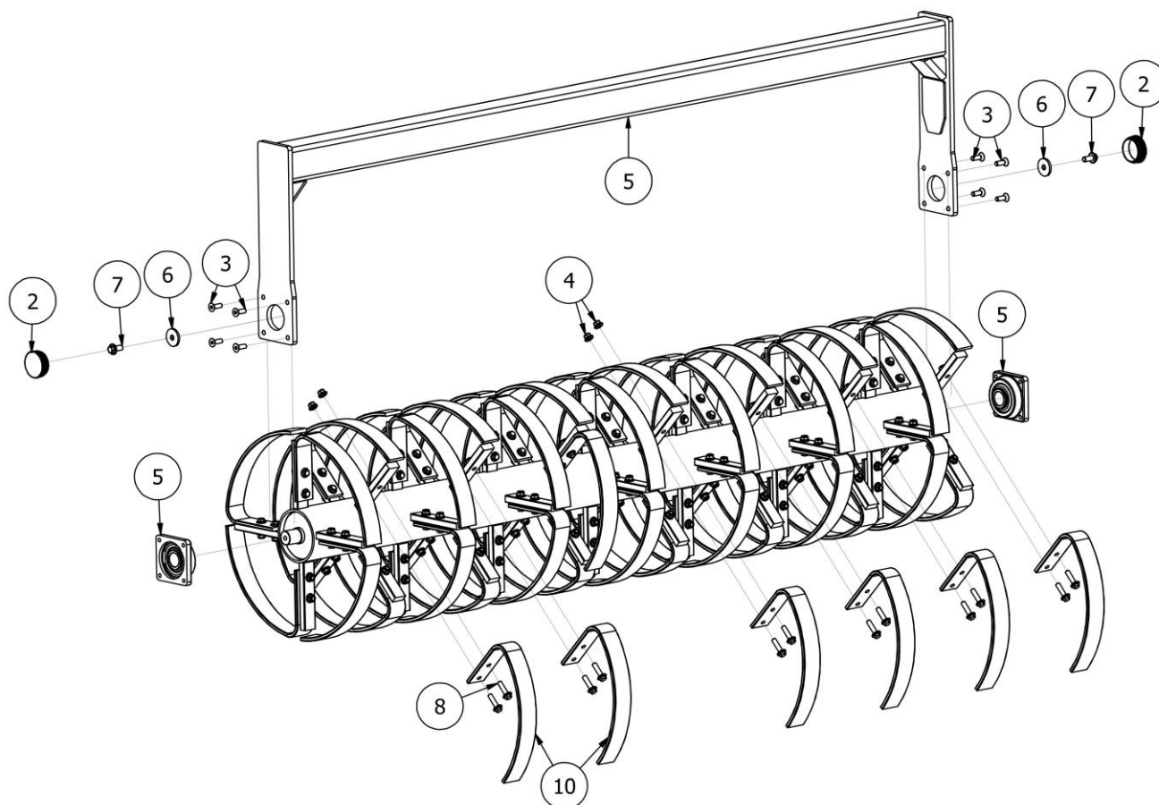
Rys. 3 EW01857-25 Wał pierścieniowy (śr. 600 mm 60x10 mm)
