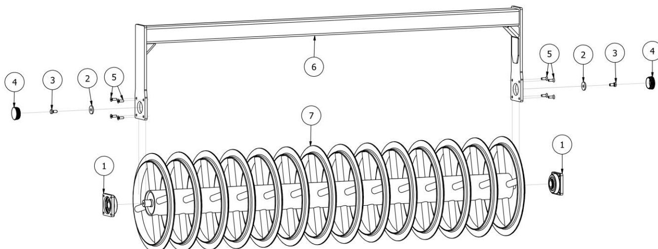
Rys. 11 EW01229-25 Wał teownikowy (śr. 600 mm) bez czyścika
