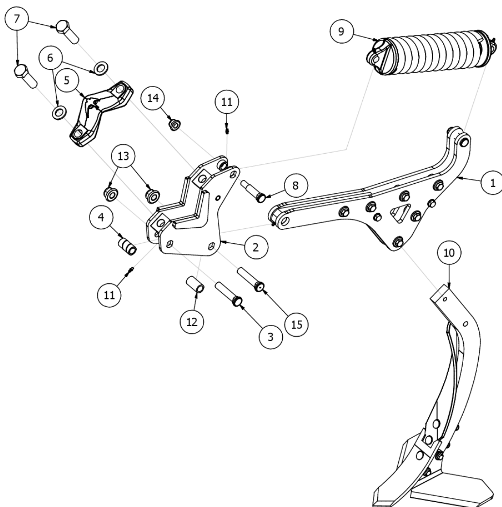
AP02975 Korpus Runner 2023 prawy zabezpieczenie sprężynowe
