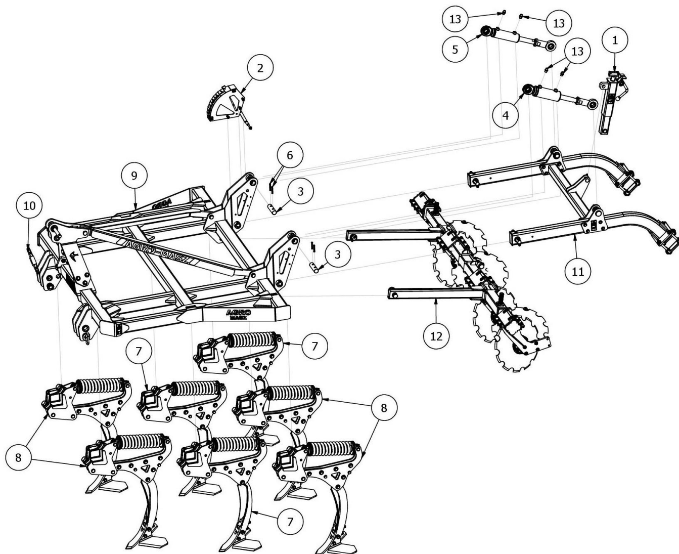
Rys. 1 A028S80B-25 RUNNER25 – podstawa maszyny
