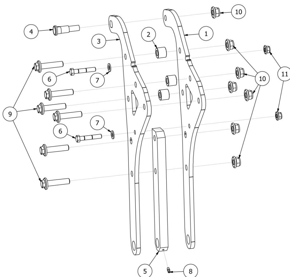
Rys. 7 AP02973 Uchwyt grzędzieli z zabezpieczeniem zrywalnym
