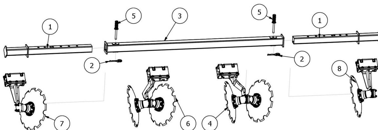
Rys. 11 AP02612 Sekcja talerzy zagarniających
