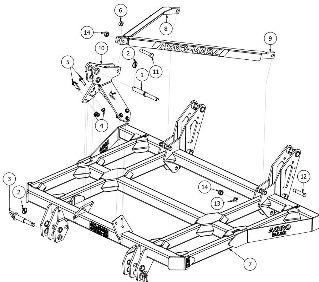
Rys. 2 AP02601 Rama kompletna RUNNER 25
