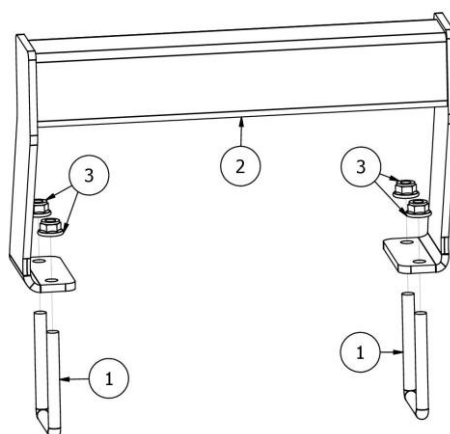
Rys. 15 SI01366 Podstawa montażowa
