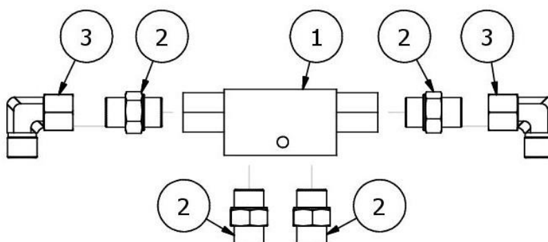
Rys. 17 HY01501 Zawór zwrotny VBPDE z przyłączkami
