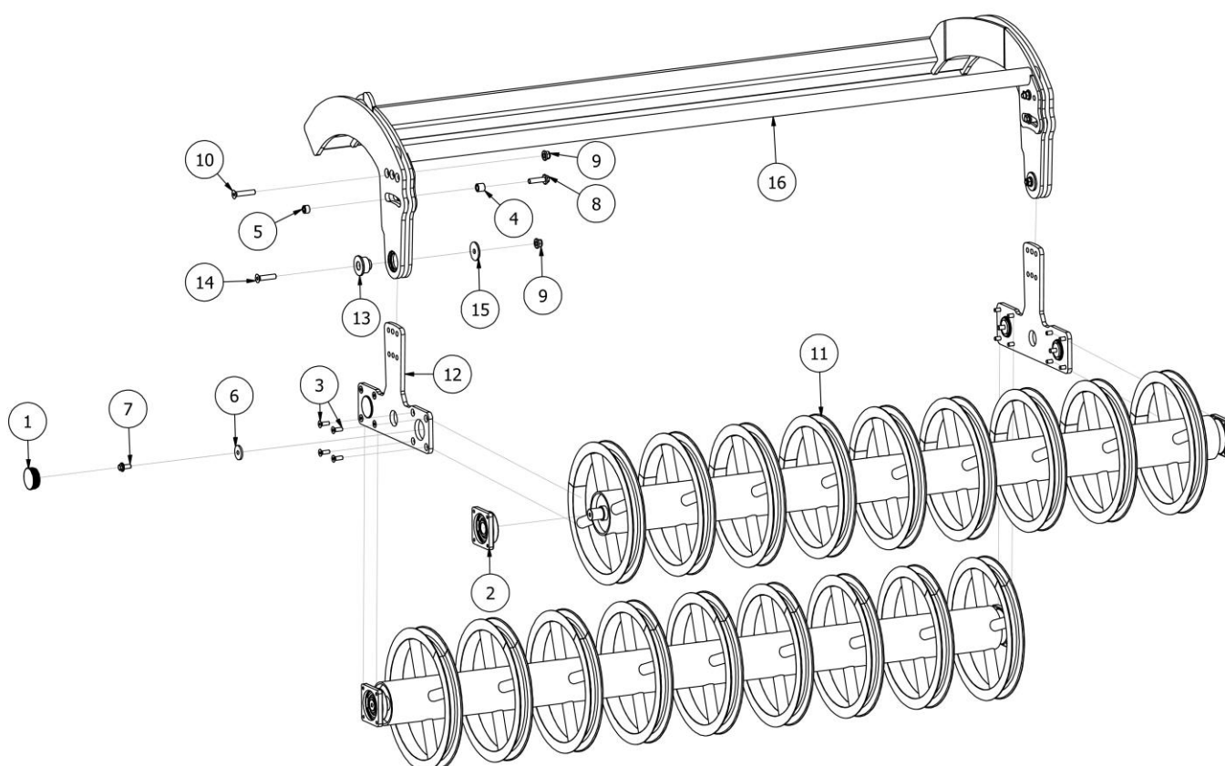
Rys. 6 EW02089-250 Wał tandem ceownikowy (2x500 mm)
