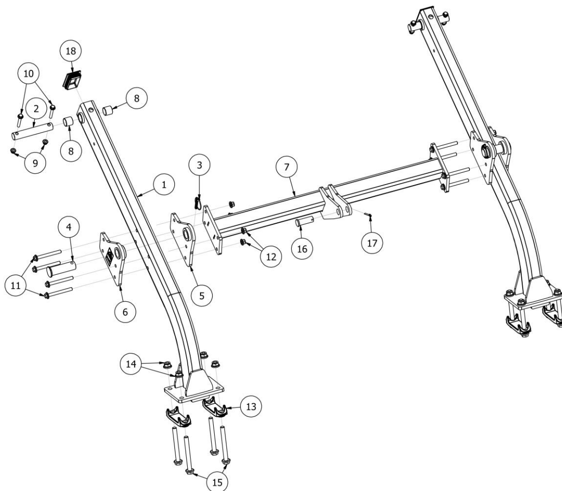
Rys. 19 AP02602 Uchwyt wału RUNNER 25
