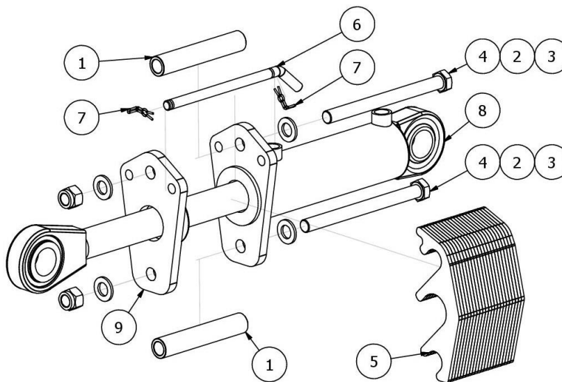
Rys. 16 EW01530 Siłownik kompletny z zapadkami 63.36.110
