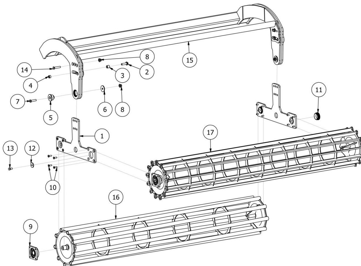
Rys. 5 EW02117-250 Wał tandem (400 mm rurowy + 400 mm strunowy)
