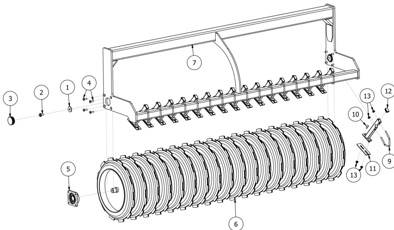
Rys. 8 EW01385-25 Wał kraker z czyścikiem (śr. 600 mm)
