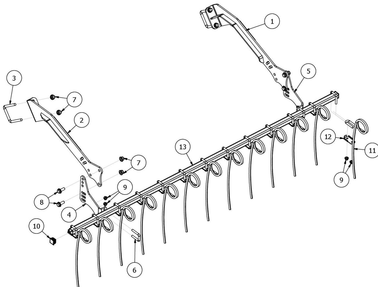
Rys. 14 EW01583-250 Zgrzebło kompletne Runner 2,5 m
