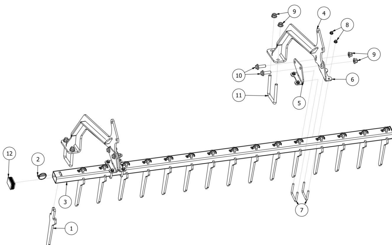
Rys. 13 EW01466-25 Czyścik palcowy wału daszkowego i teownikowego
