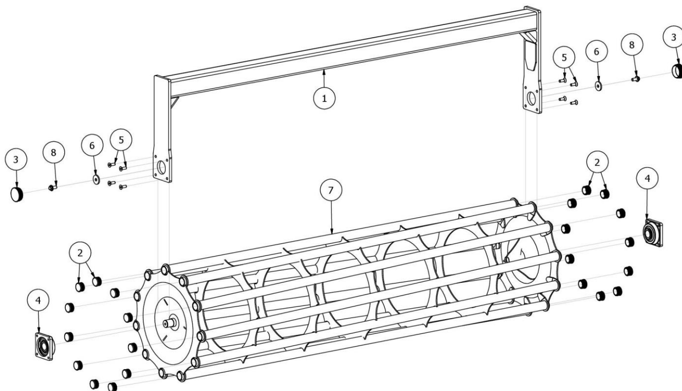
Rys. 2 EW00100-250 Wał rurowy 600 (2.5 m)
