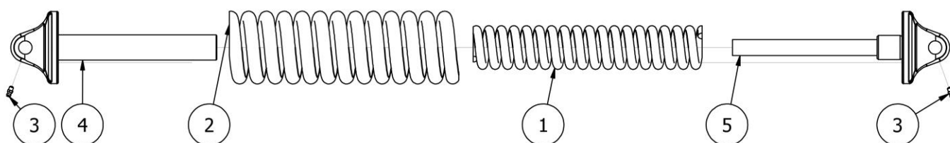
Rys. 5 AP01075 Sprężyna zabezpieczająca kompletna (RUNNER)
