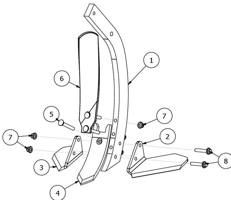
Rys. 9 AP03067 Grządziel lewa kompletna
