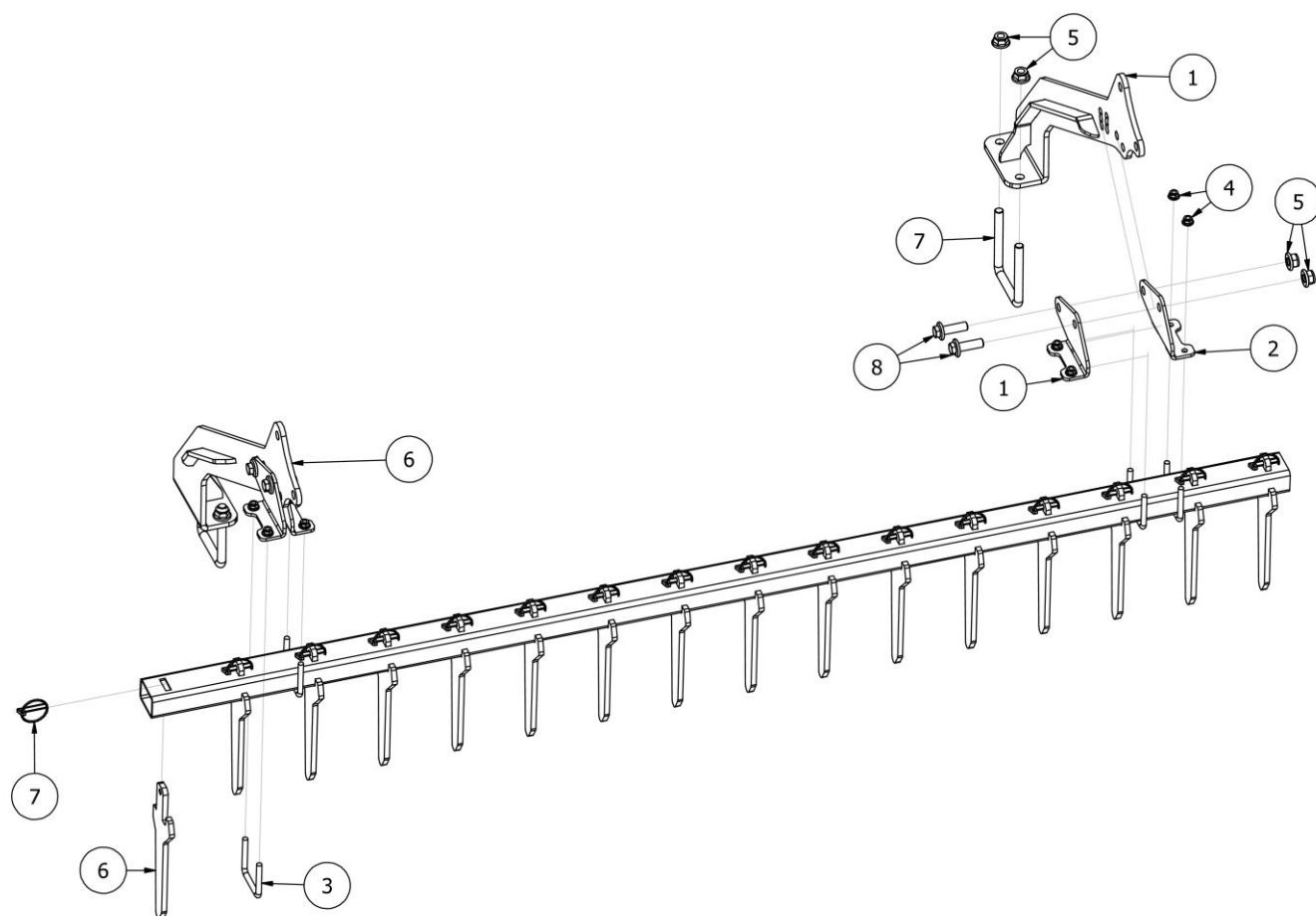
Rys. 4 EW01807-25 Czyścik palcowy wału pierścieniowego (śr. 600 mm 60x10 mm)
