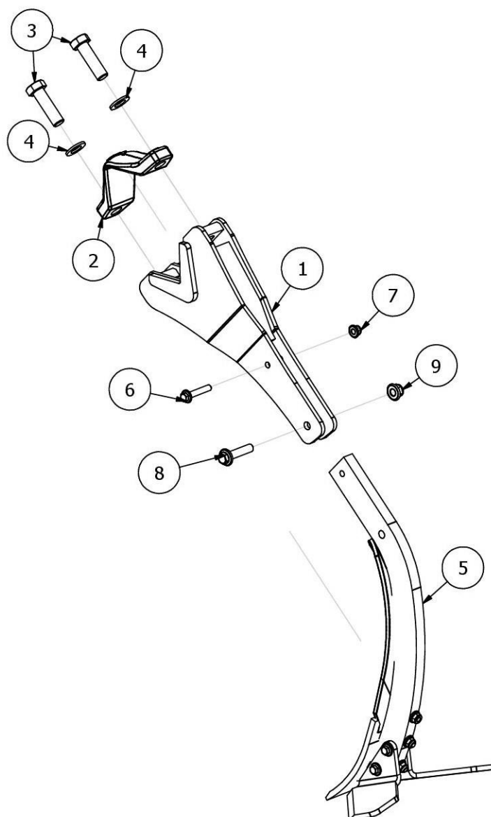
Rys. 8 AP03080 Korpus zrywalny lewy RUNNER
