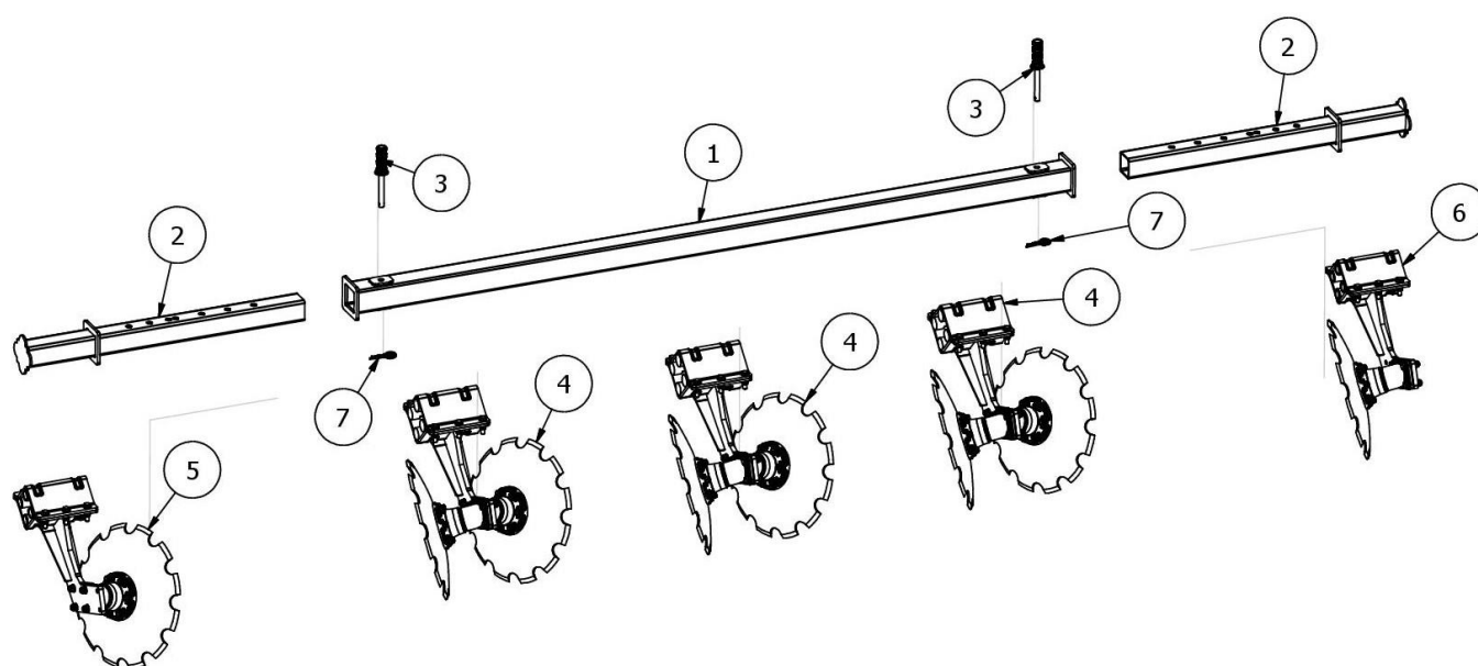
Rys. 11 AP03065 Sekcja talerzy zagarniających
