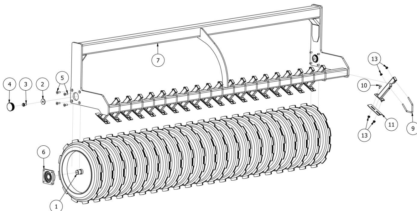
Rys. 27 EW01385-30 Wał kraker z czyścikiem (śr. 600 mm)
