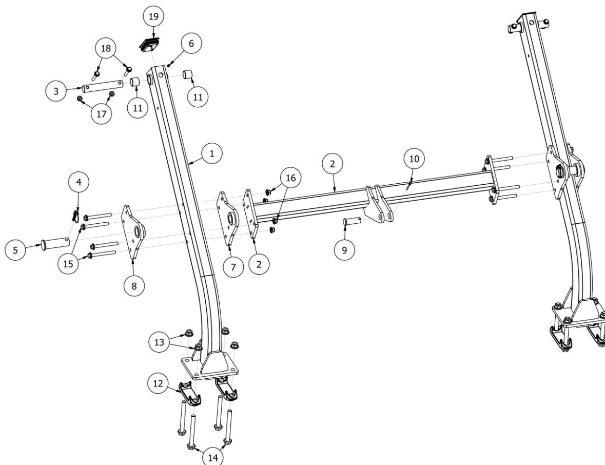
Rys. 18 AP02283 Uchwyt kompletny wału
