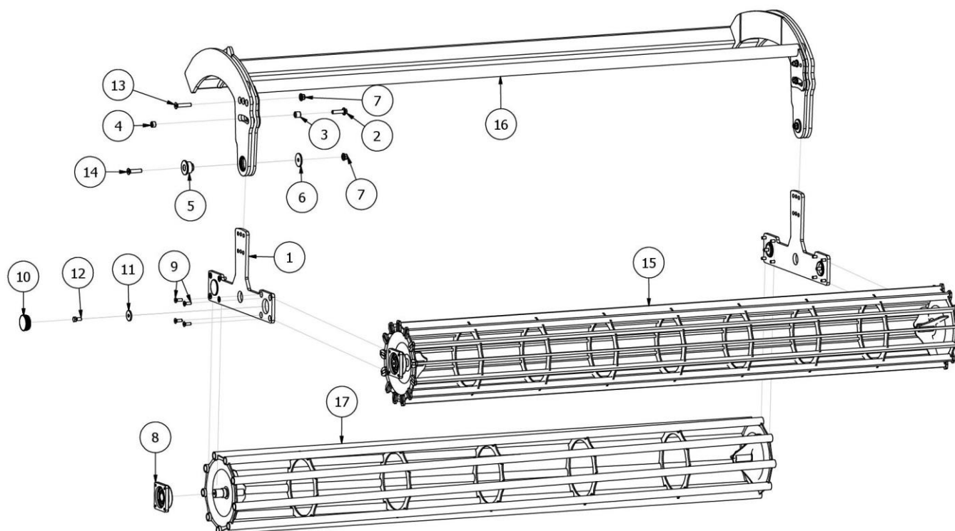
Rys. 24 EW02117-300 Wał tandem (400 mm rurowy + 400 mm strunowy)
