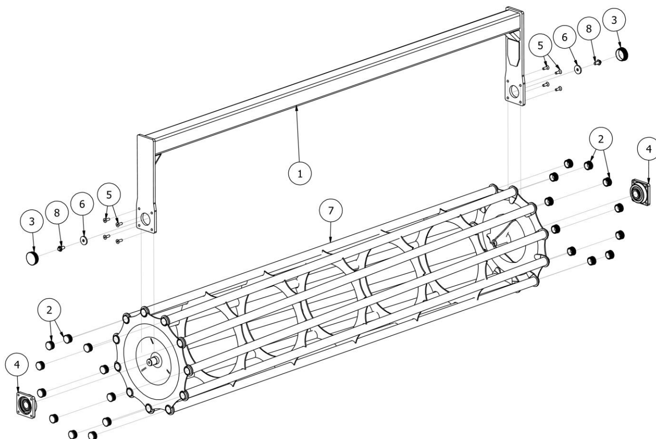
Rys. 20 EW00100-300 Wał rurowy 600 (3.0 m)
