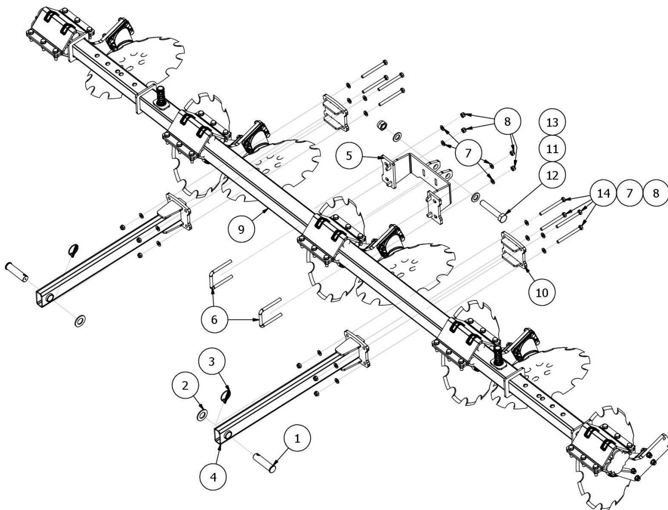
Rys. 10 AP03064 Rama talerzy zagarniających (RUNNER)
