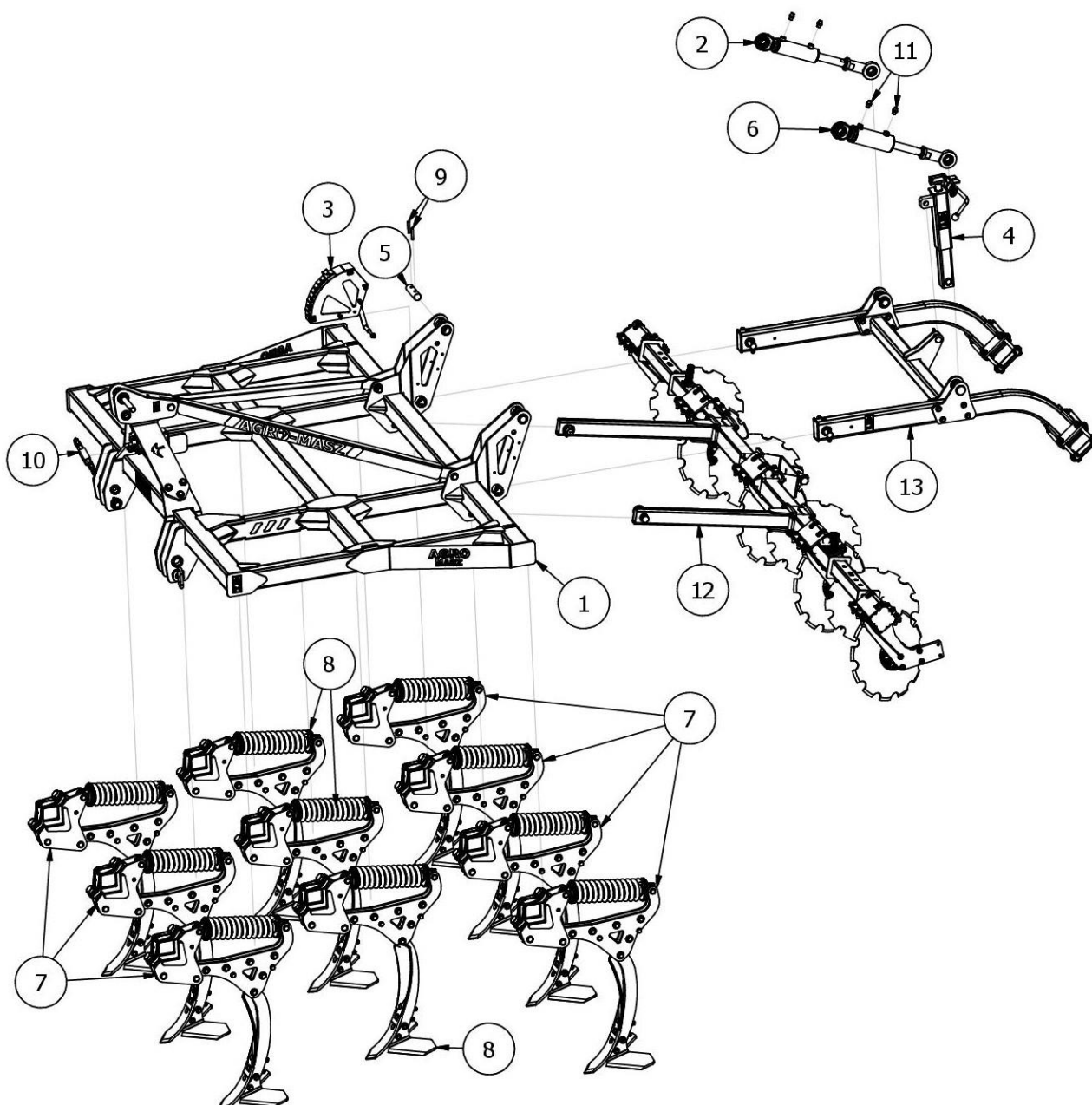
Rys. 1 A028S80B-30 RUNNER30 – podstawa maszyny
