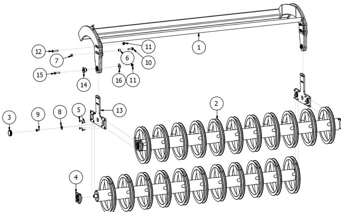
Rys. 25 EW02089-300 Wał tandem ceownikowy (2x500 mm)
