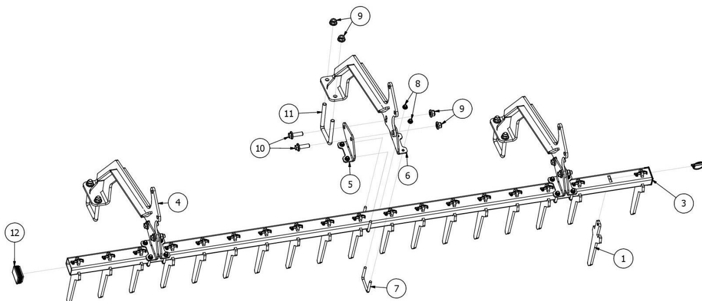
EW01466-30 Czyścik palcowy wału daszkowego i teownikowego
