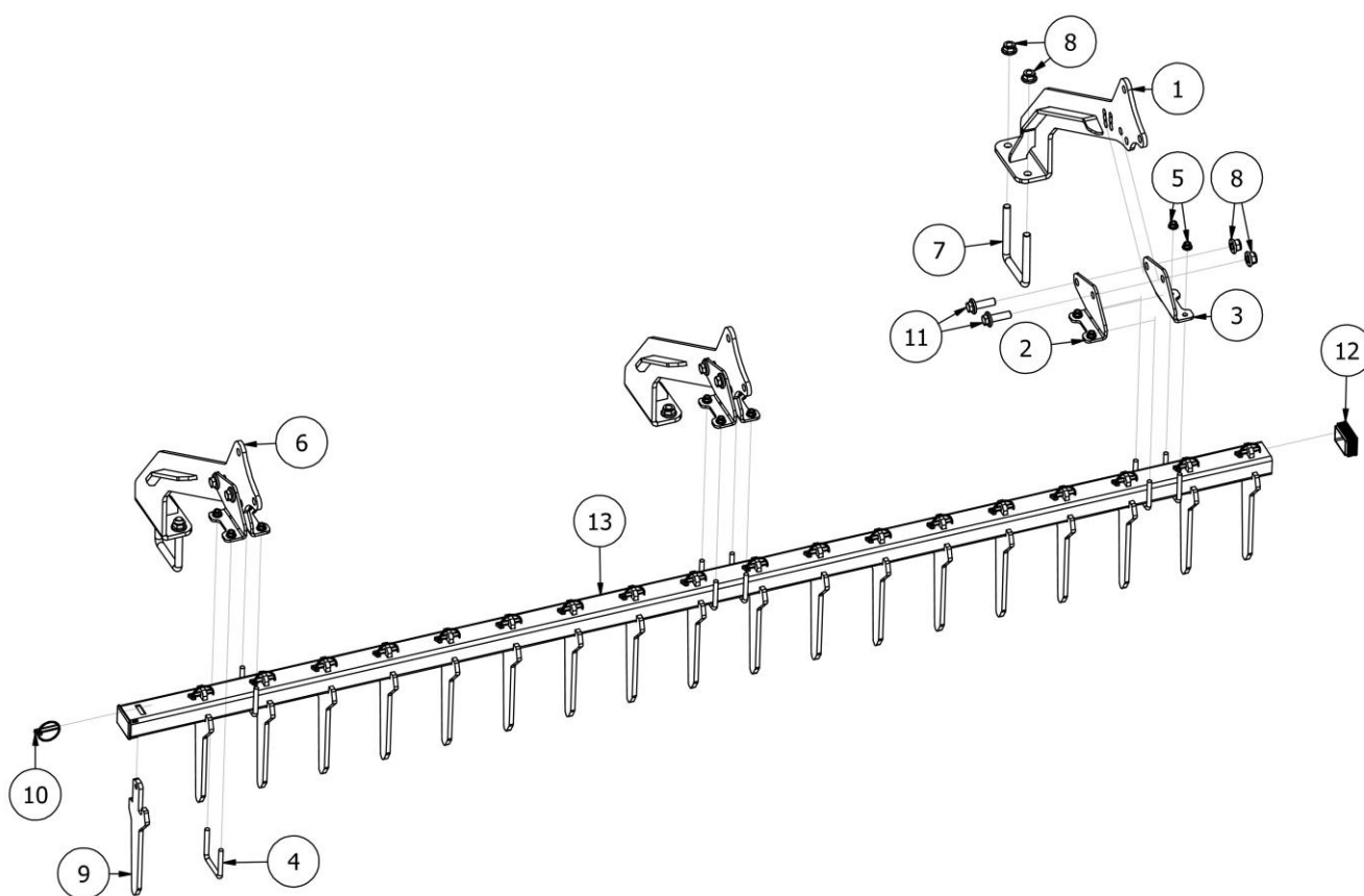
Rys. 22 EW01807-30 Czyścik palcowy wału pierścieniowego
