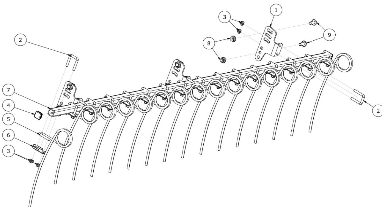
EW01582-30 Zgrzebło za wałem pojedynczym 3m
