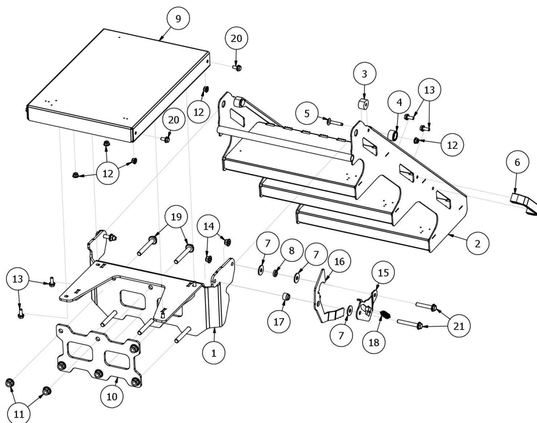
Rys. 37 AP02848 Stopnie kompletne
