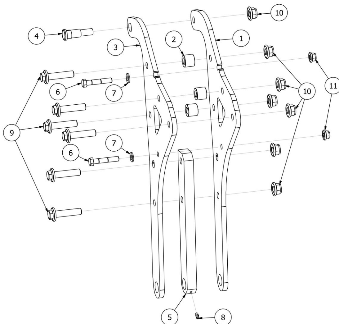
Rys. 7 AP02973 Uchwyt grądzeli z zabezpieczeniem zrywalnym
