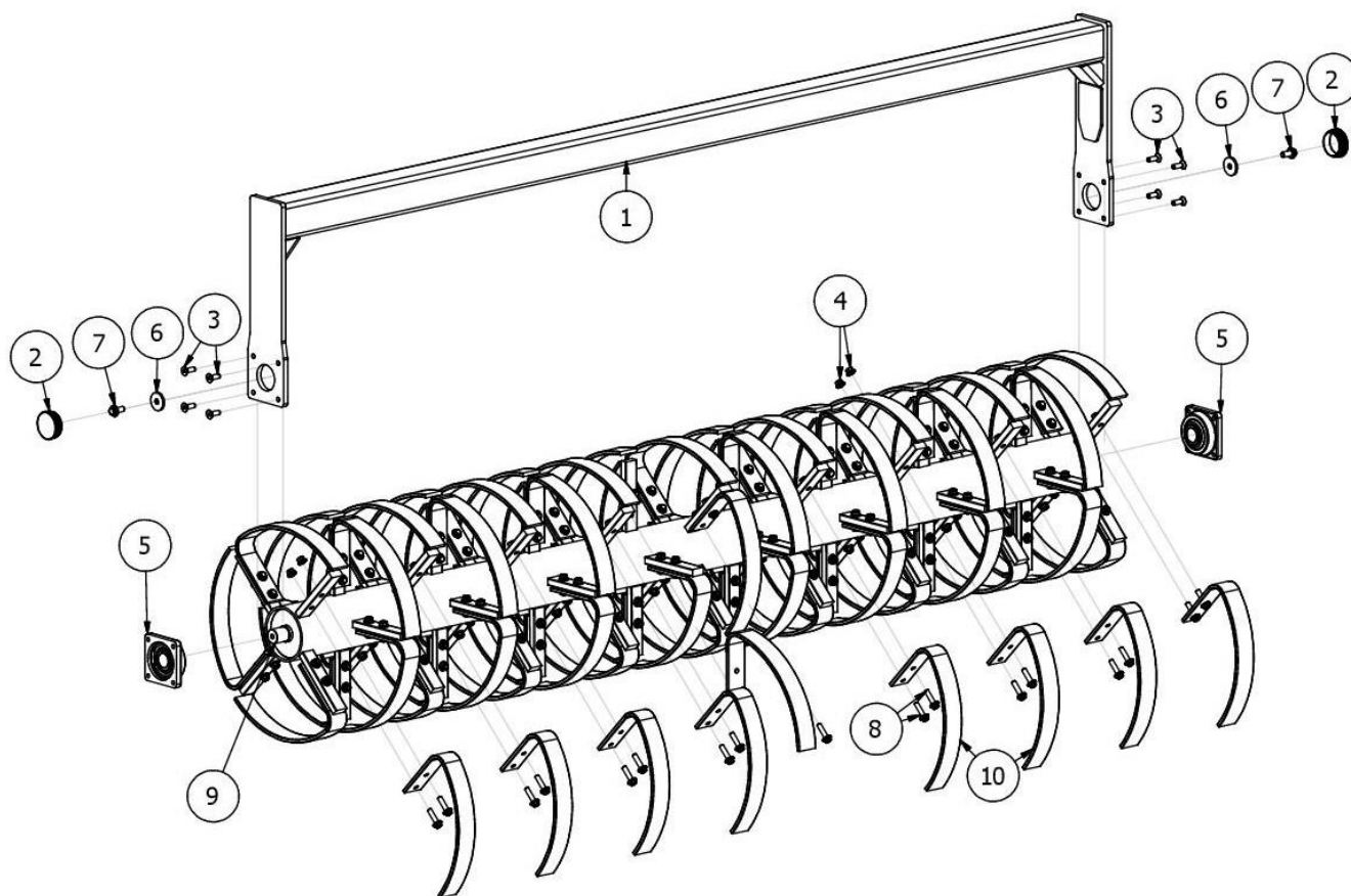
Rys. 21 EW01857-30 Wał pierścieniowy 3,0 m (śr. 600 mm 60x10 mm)
