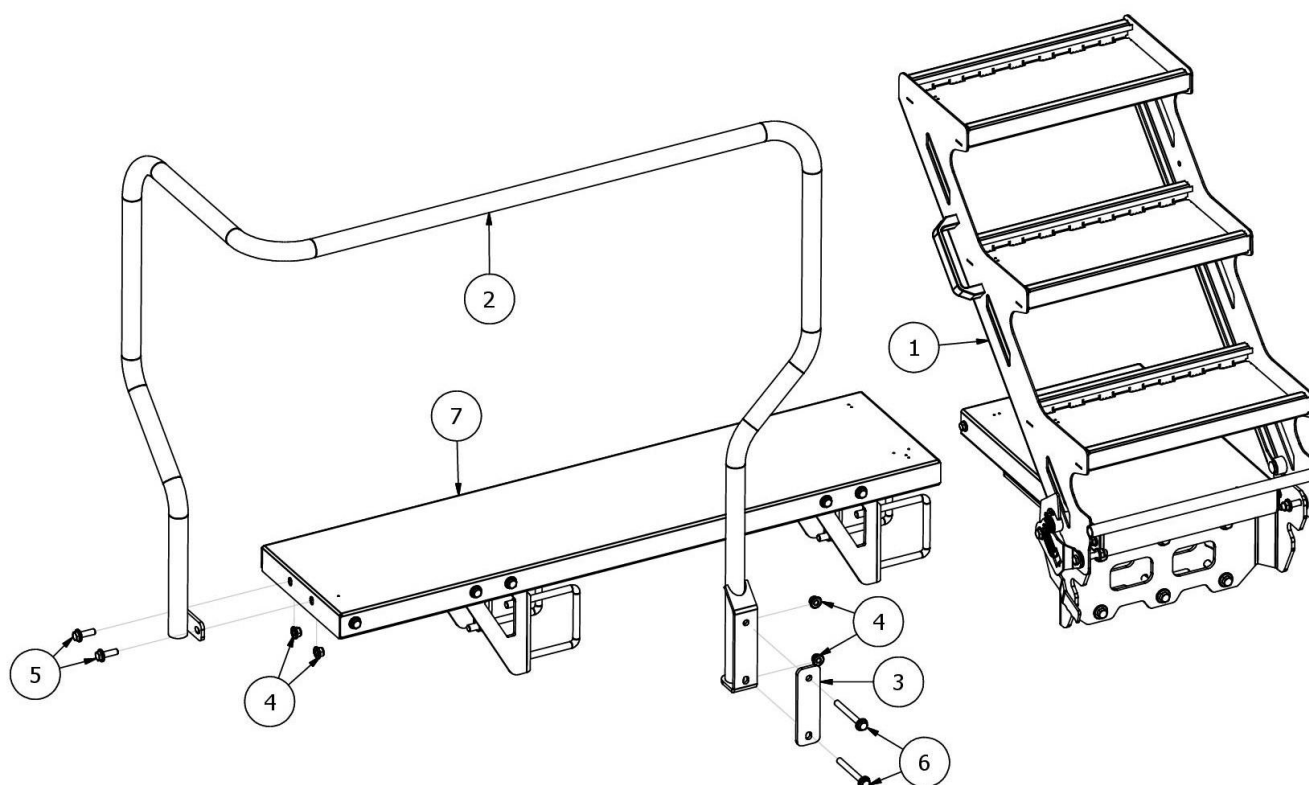
Rys. 35 AP02864 Schody z podestem i barierką Runner 30
