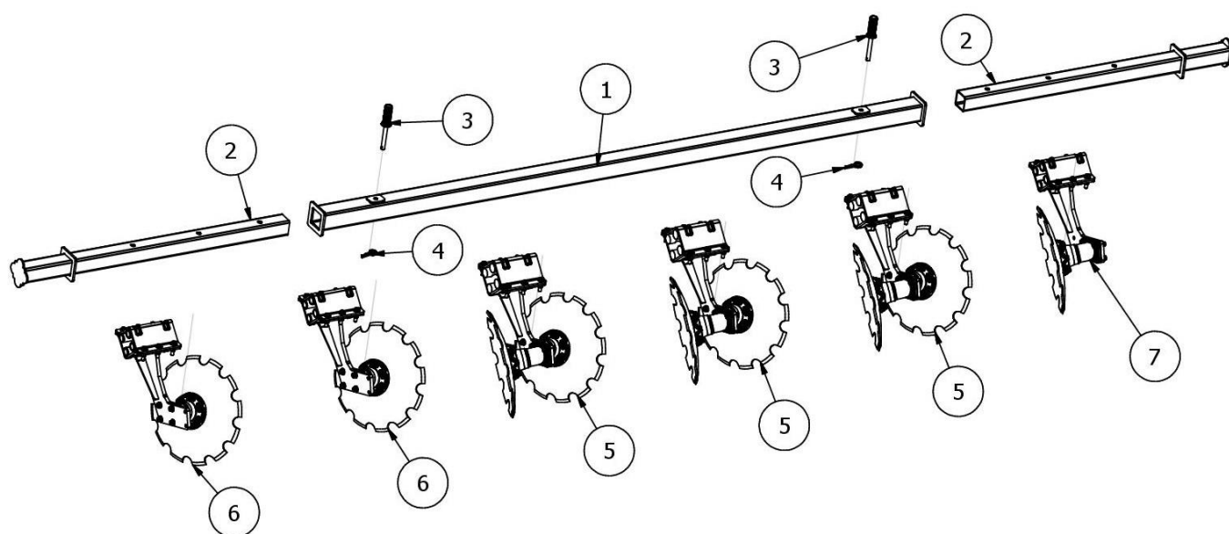
Rys. 11 AP03104 Sekcja talerzy zagarniających 3,5m
