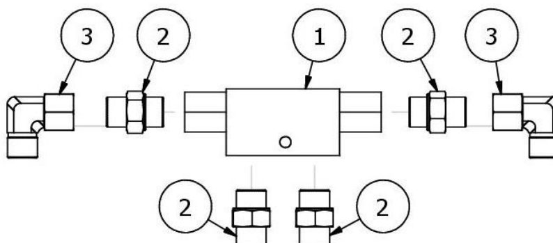
Rys. 16 HY01501 Zawór zwrotny VBPDE z przyłączkami
