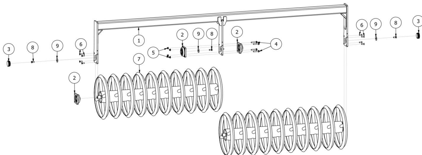
EW01228-35 Wał daszkowy (śr. 600 mm) bez czyścika
