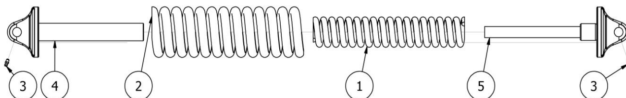
Rys. 5 AP01075 Sprężyna zabezpieczająca kompletna (RUNNER)
