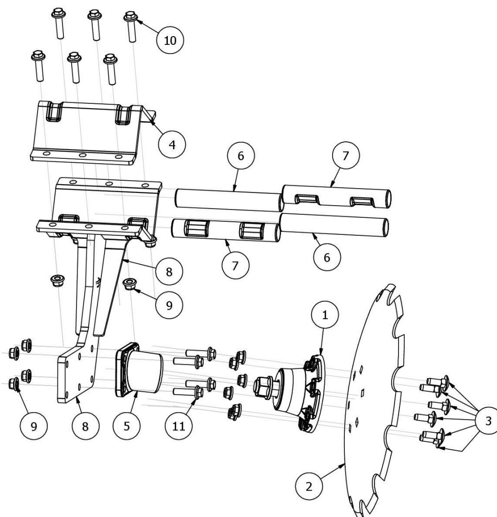
Rys. 14 AP02506-05 Noga lewa kompletna z talerzem 460 "C" wraz z mocowaniem do ramy
