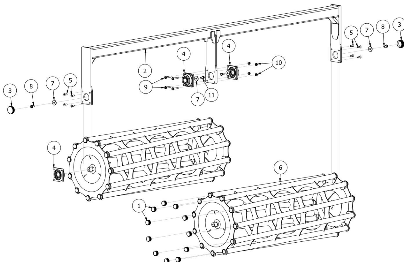
Rys. 22 EW00100-350 Wał rurowy 600 (3.5 m)
