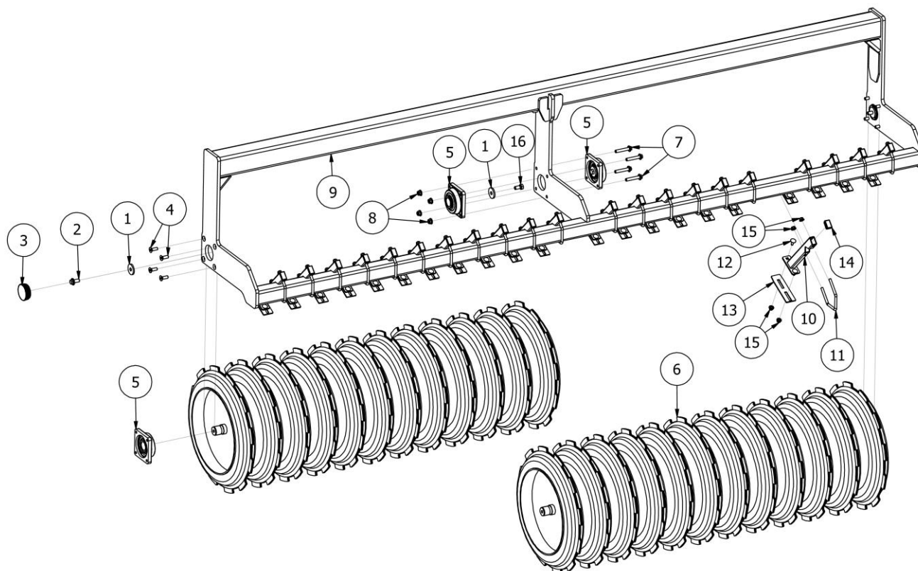
Rys. 27 EW01385-35 Wał kraker z czyścikiem (śr. 600 mm)
