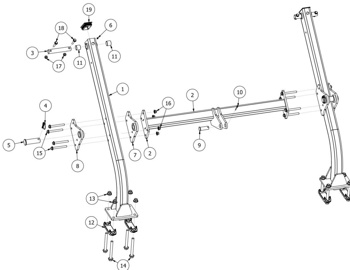
Rys. 20 AP02283 Uchwyt kompletny wału
