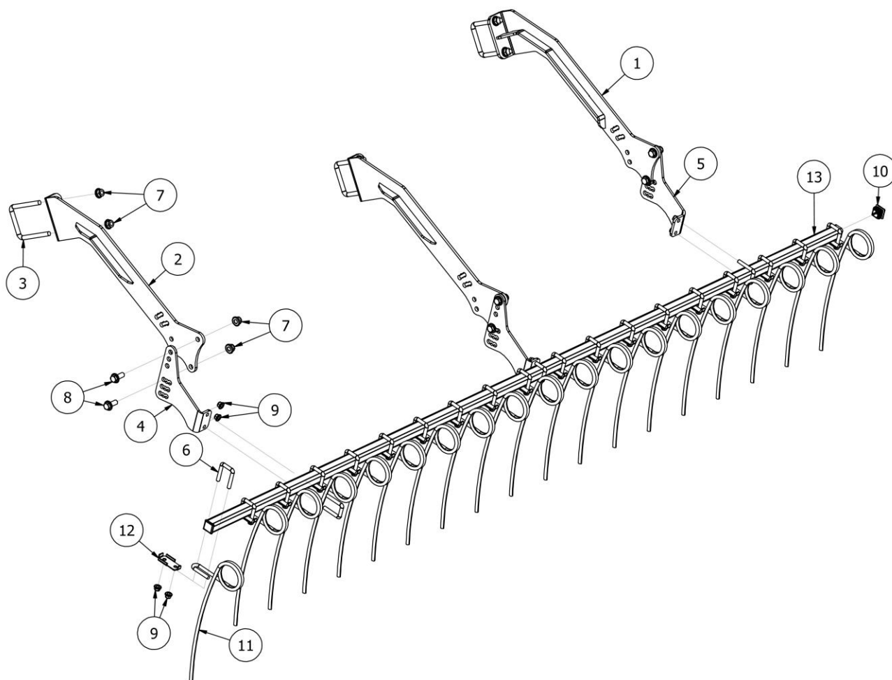
EW01583-350 Zgrzebło kompletne Runner 3,5 m
