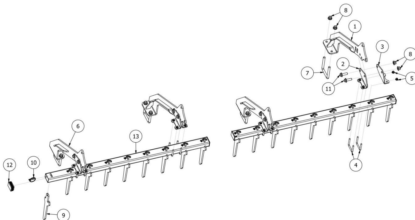
Rys. 24 EW01807-35 Czyścik palcowy wału pierścieniowego (śr. 600 mm 60x10 mm)
