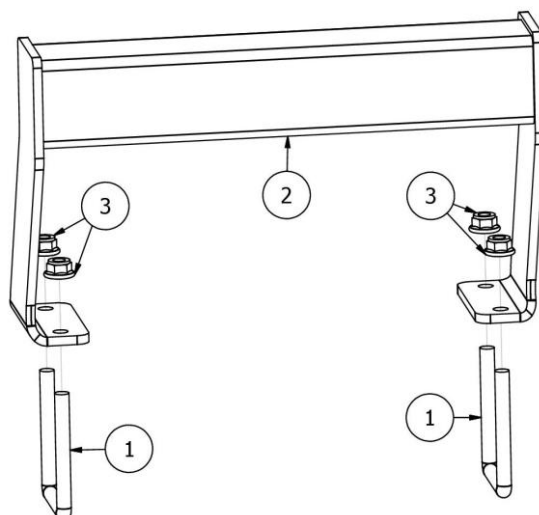
SI01366 Podstawa montażowa
