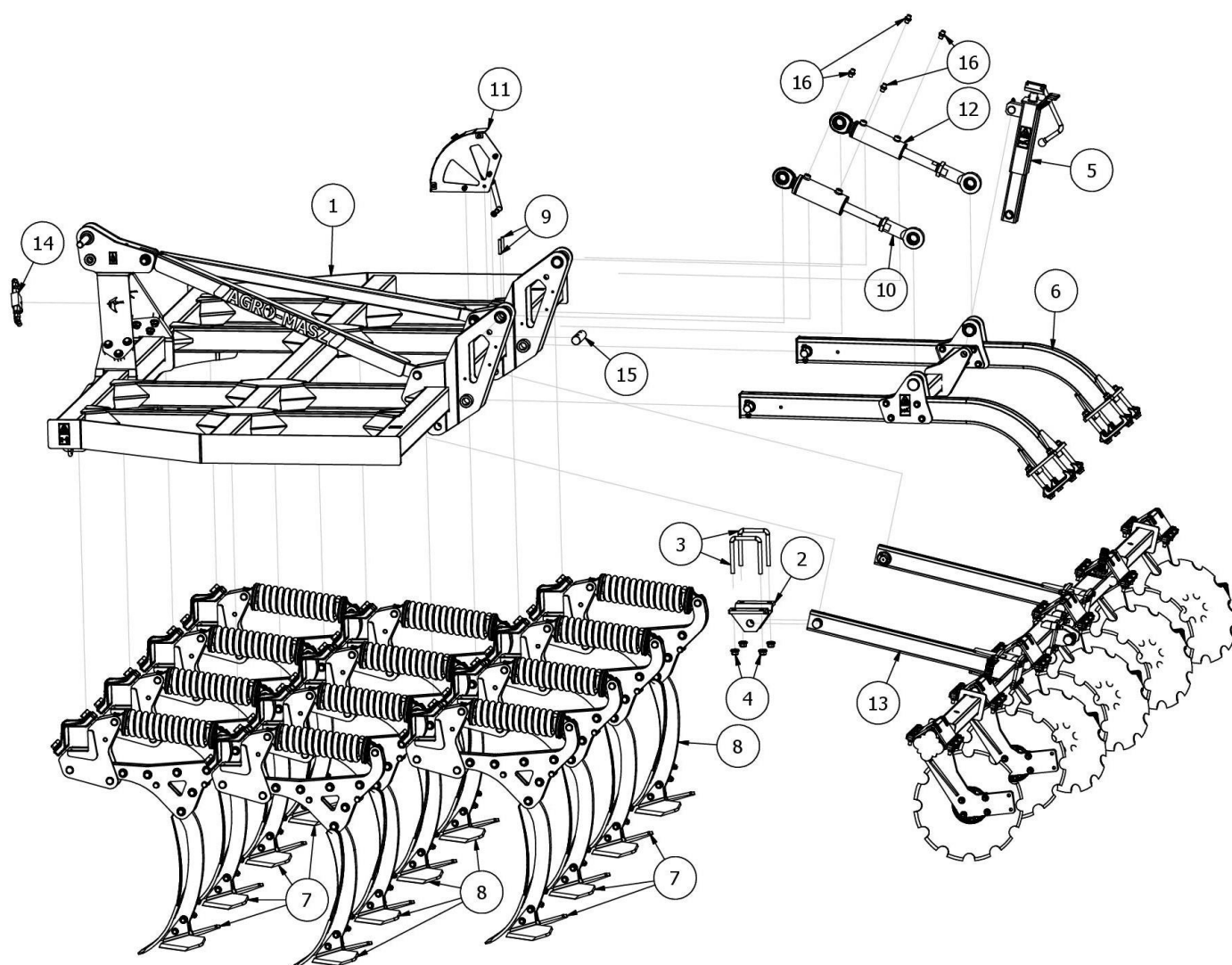
Rys. 1 A028S80B-35 RUNNER35 – podstawa maszyny
