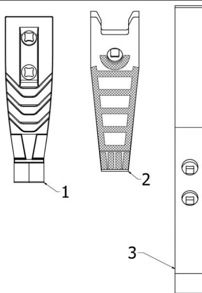
Rys. 36 Opcjonalne dłuta
