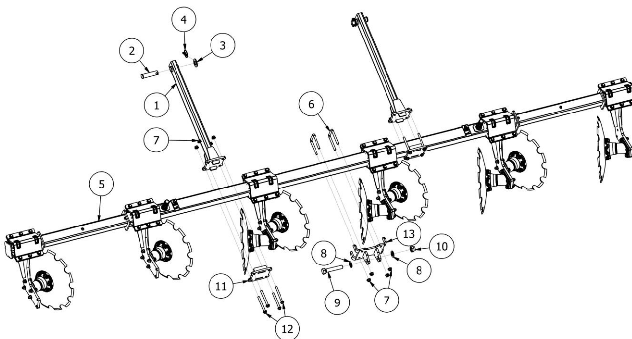
Rys. 10 AP03103 Rama talerzy zagarniających Runner 3,5
