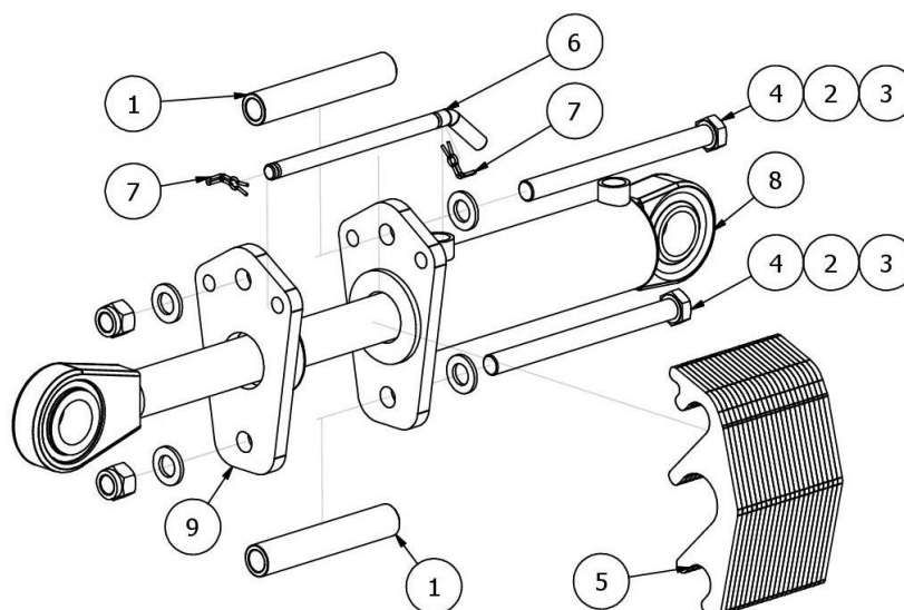
EW01530 Siłownik kompletny z zapadkami 63.36.110
