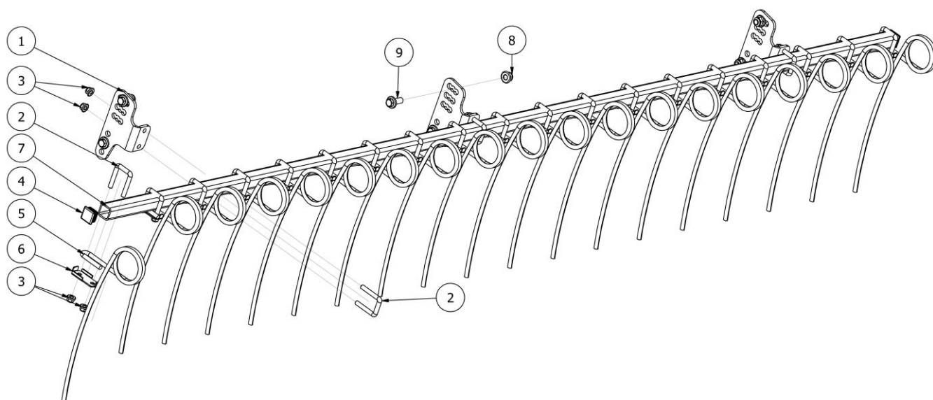
EW01582-350 Zgrzebło kompletne Runner 3,5 m
