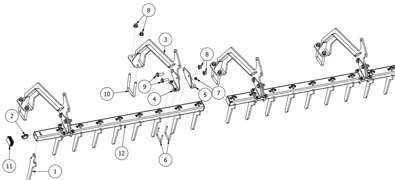
EW01466-35 Czyścik palcowy wału daszkowego i teownikowego
