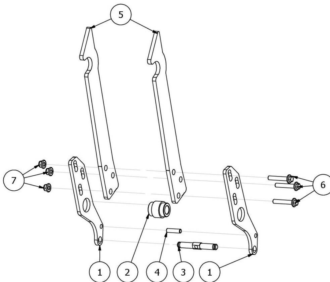
AP01379 Zabezpieczenie Transportowe
