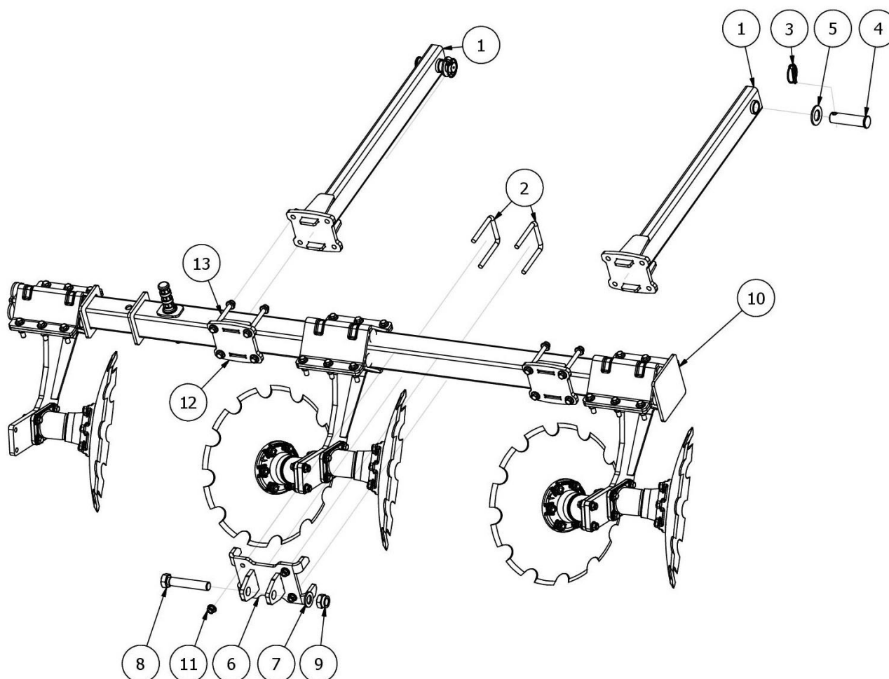
AP01624 Rama lewa z talerzami zagarniającymi
