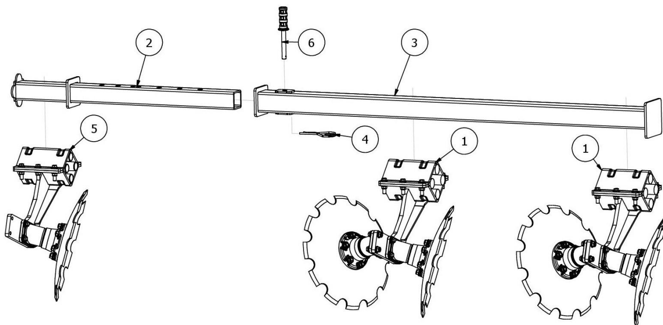
Rys. 13 AP01350 Sekcja lewa talerzy zagarniających
