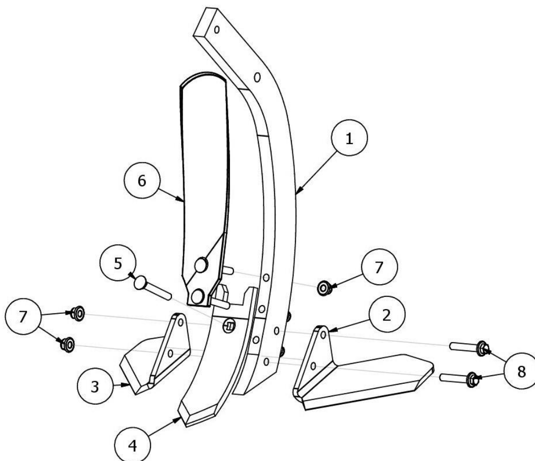
AP03067 Grządziel lewa kompletna
