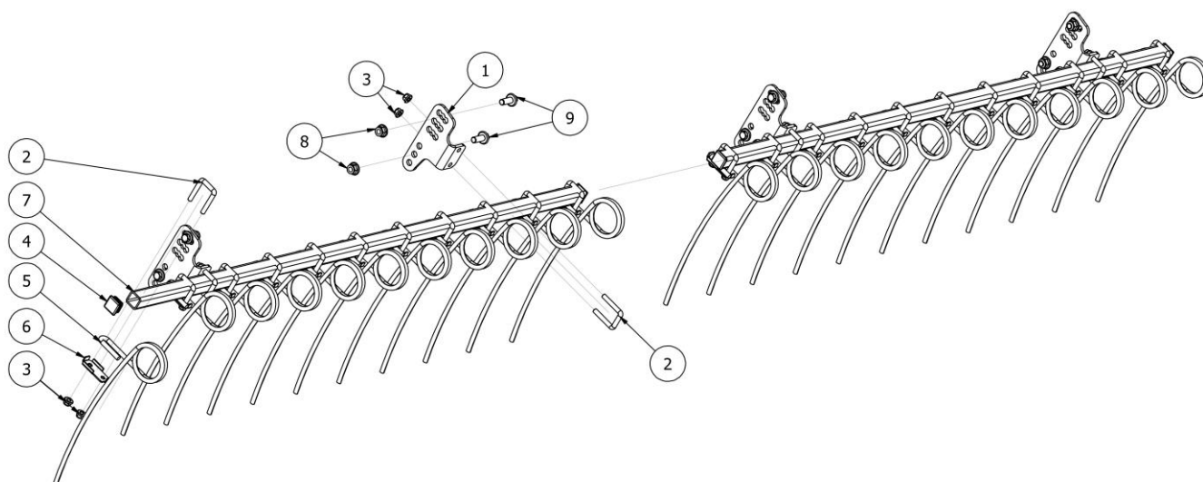
EW01582-H40 Zgrzebło za wałem pojedynczym (wymaga czyścika palcowego)
