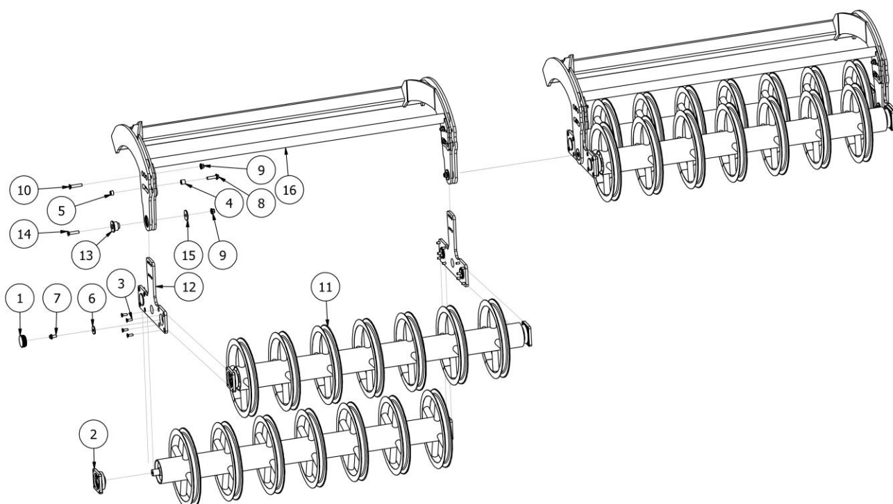
EW02089-H400 Wał tandem ceownikowy (2x500 mm)
