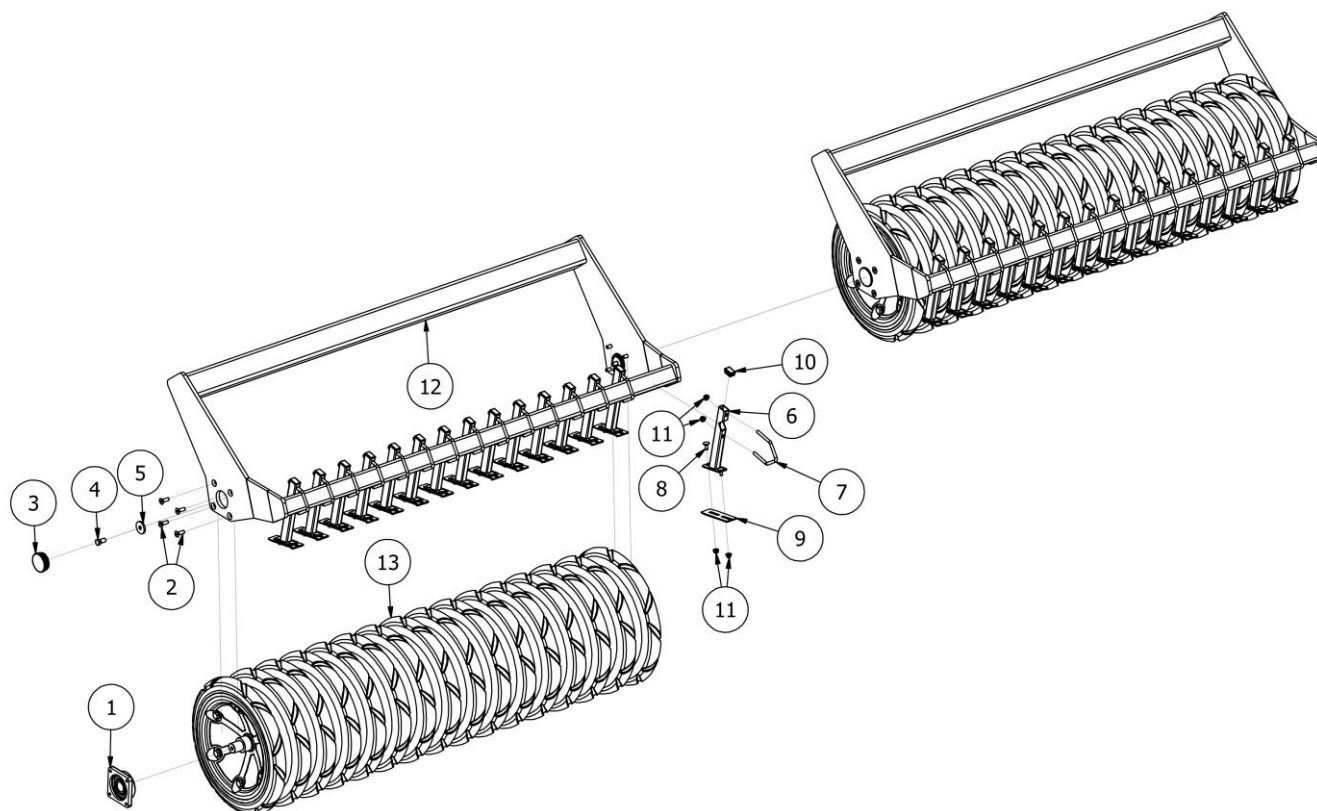
EW02103-H400 Wał gumowy z czyścikiem (śr. 560 mm) wersja 2020
