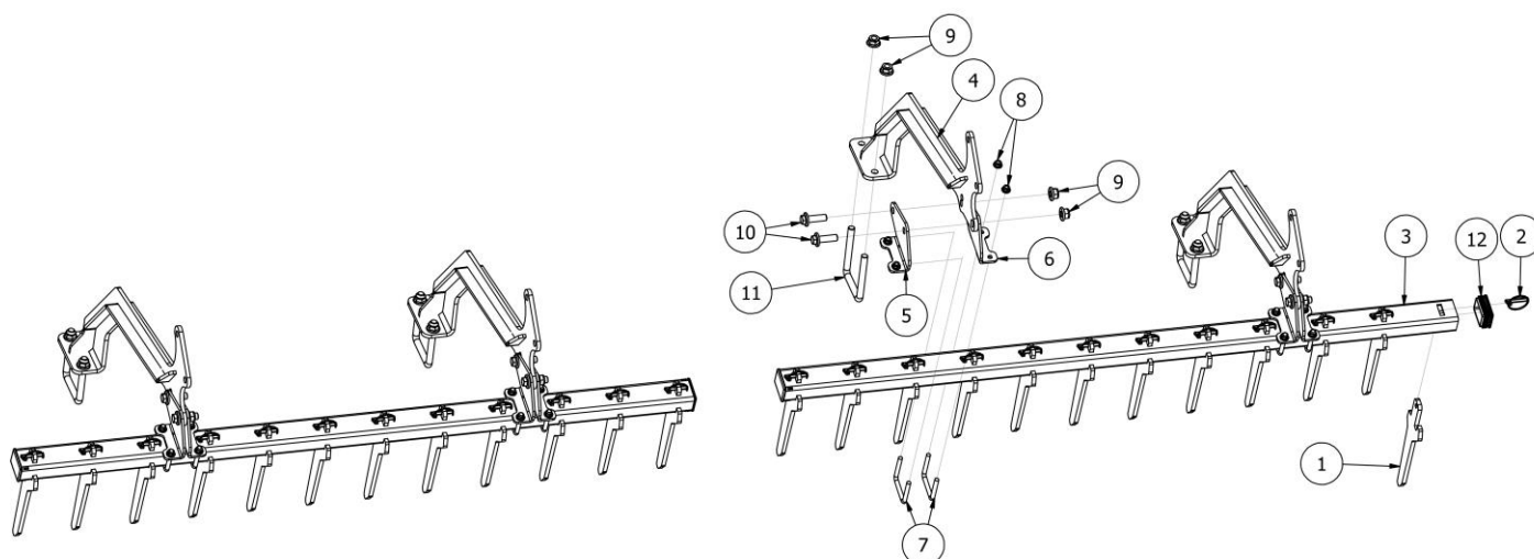
EW01466-H40 Czyścik palcowy wału daszkowego i teownikowego
