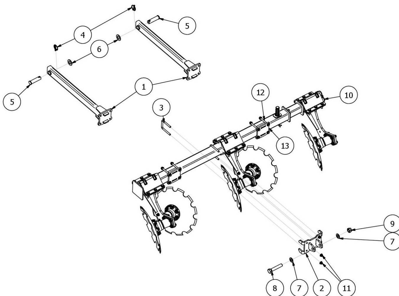
AP01626 Rama prawa z talerzami zagarniającymi
