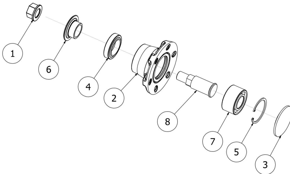
Rys. 34 EW00128 Piasta bezobsługowa kompletna 2010 (AT, BT)
