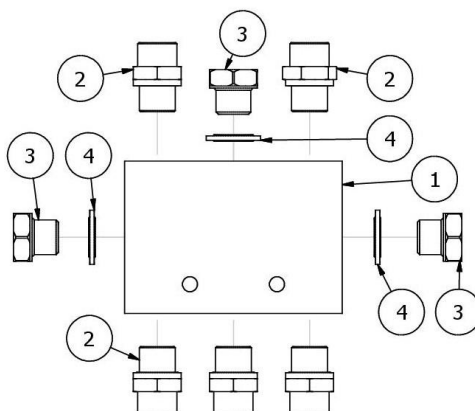
HY01493 Rozdzielacz z przyłączkami
