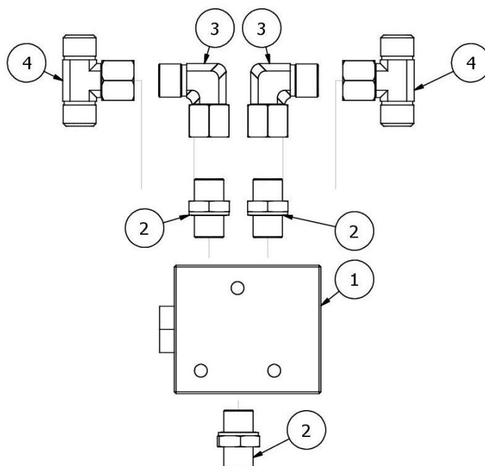
HY01492 Dzielnik strumienia kompletny z przyłączkami
