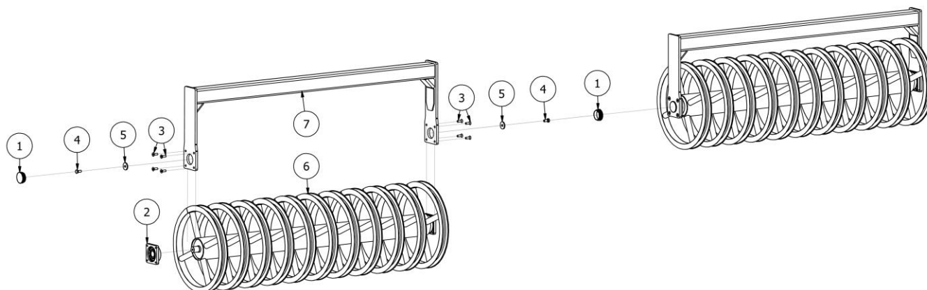
EW02708-H40 wał ceownikowy (śr. 600 mm) bez czyścika
