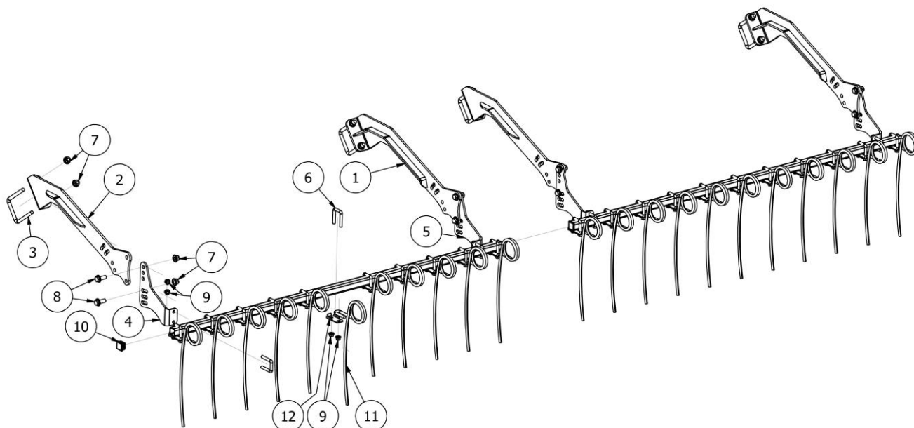
EW01583-H40 Zgrzebło za wałem pojedynczym (nie wymaga czyścika palcowego)
