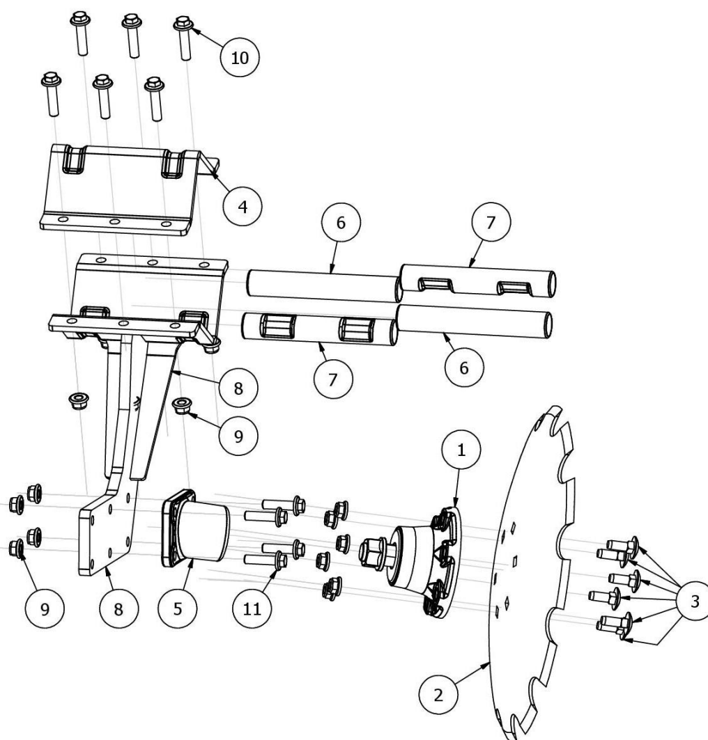
Rys. 18 AP02506-05 Noga lewa kompletna z talerzem 460 "C" wraz z mocowaniem do ramy
