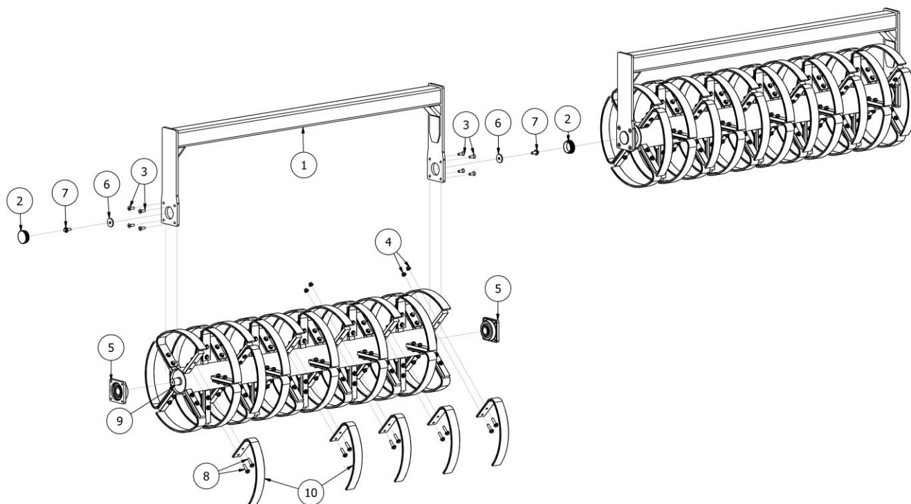
EW01857-H40 Wał pierścieniowy (śr. 600 mm 60x10 mm)
