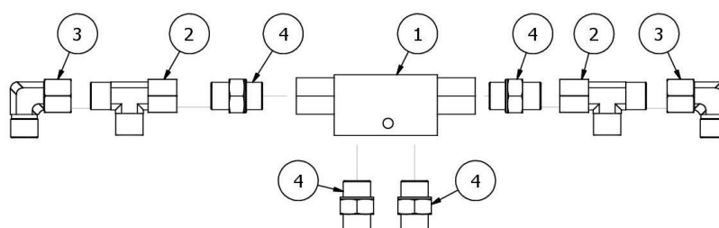
Rys. 35 HY01495 Zawór zwrotny VBPDE z przyłączkami
