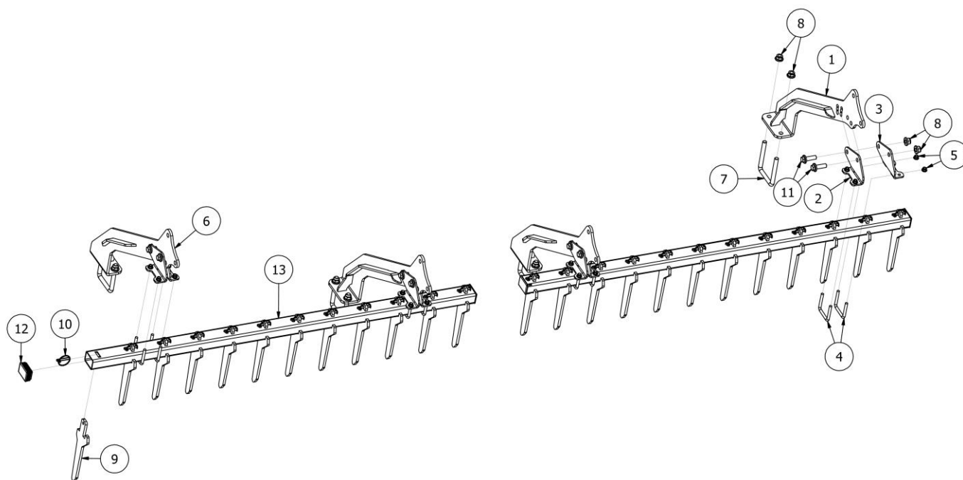
EW01807-H40 Czyścik palcowy wału pierścieniowego (śr. 600 mm 60x10 mm)
