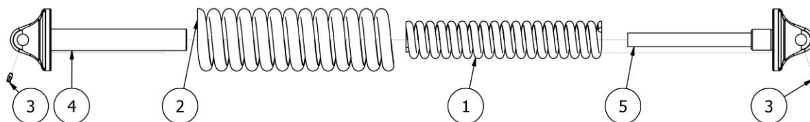
Rys. 6 AP01075 Sprężyna zabezpieczająca kompletna (RUNNER)
