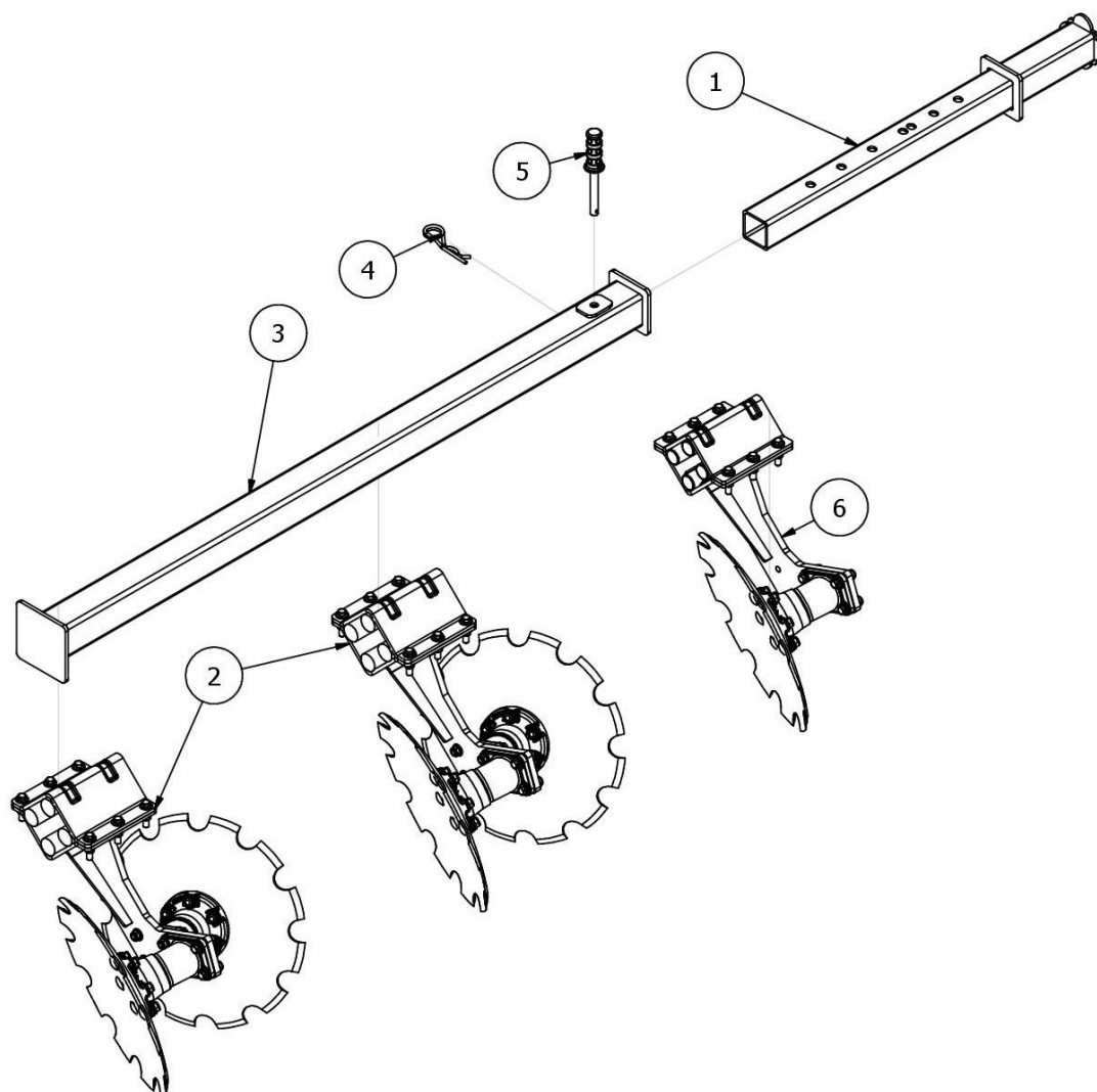
AP01625 Sekcja prawa talerzy zagarniających
