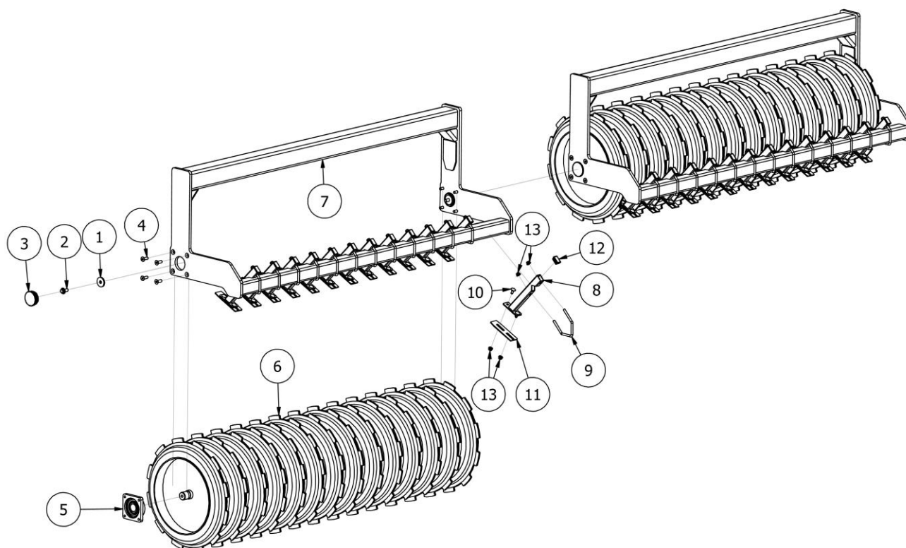
EW01385-H40 Wał kraker z czyścikiem (śr. 600 mm)
