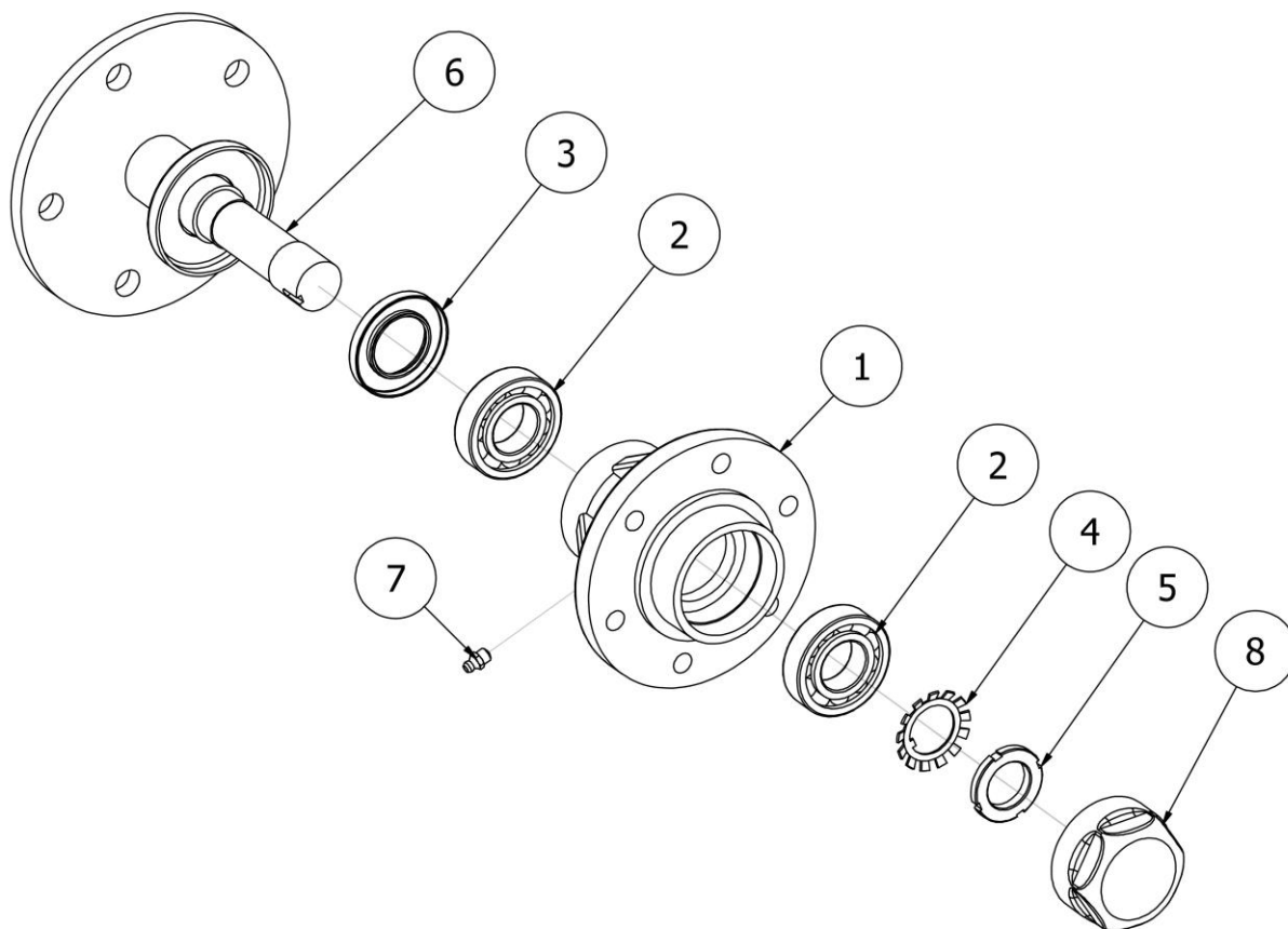
Rys. 7 SI00484 Piasta kompletna SR300 nienapędowa
