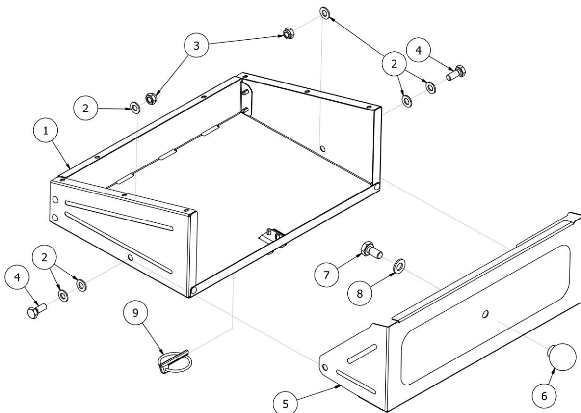
Rys. 12 SI01645 Skrzynka narzędziowa
