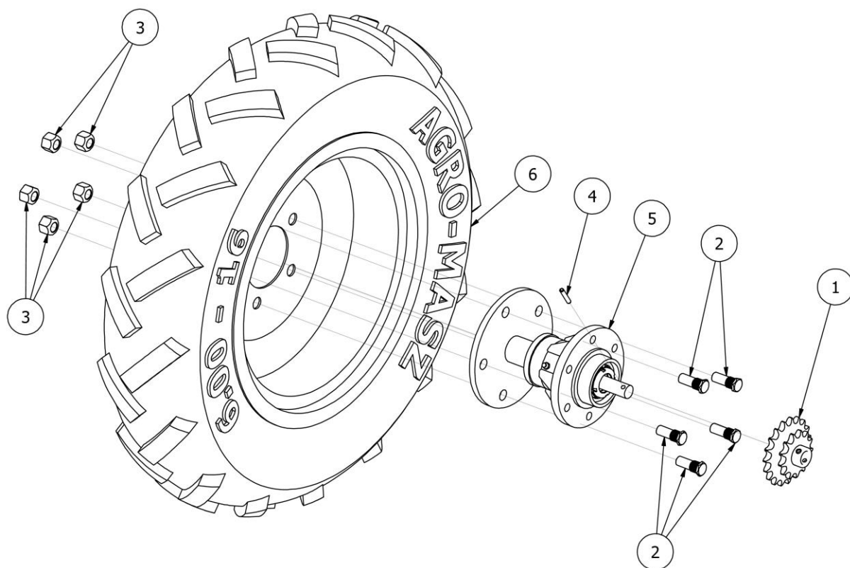
Rys. 4 PL00385 Koło kompletne SR (napędowe)
