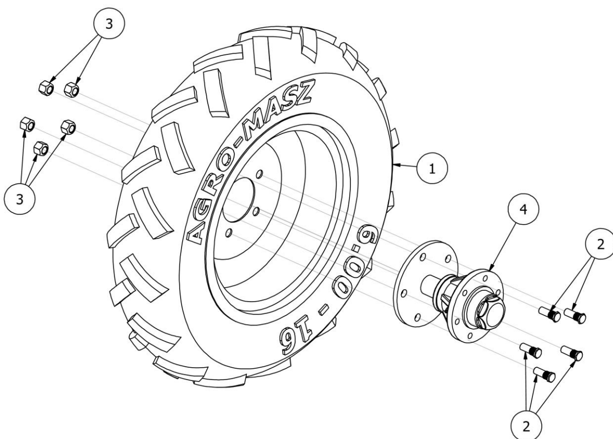
Rys. 6 SI00482 Koło kompletne SR (nienapędowe)
