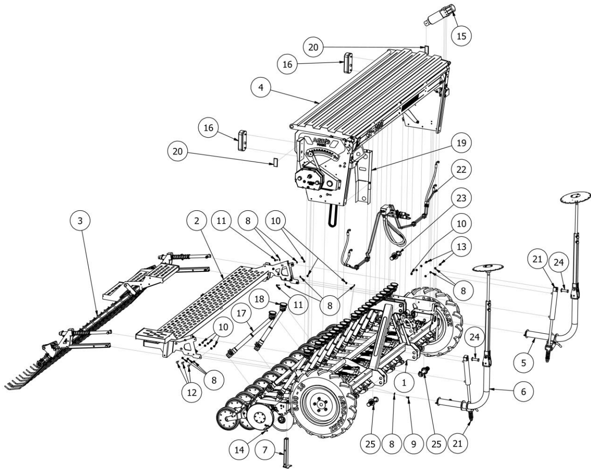
S012TC Siewnik SR300T 2016, talerz czyszczący
