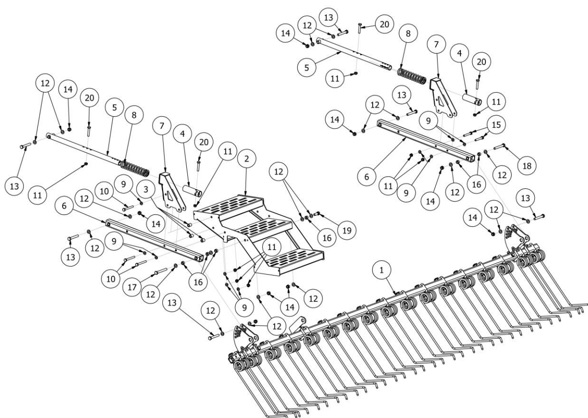
Rys. 14 SI02150 Zagarniacz SR300 2016, kompletny
