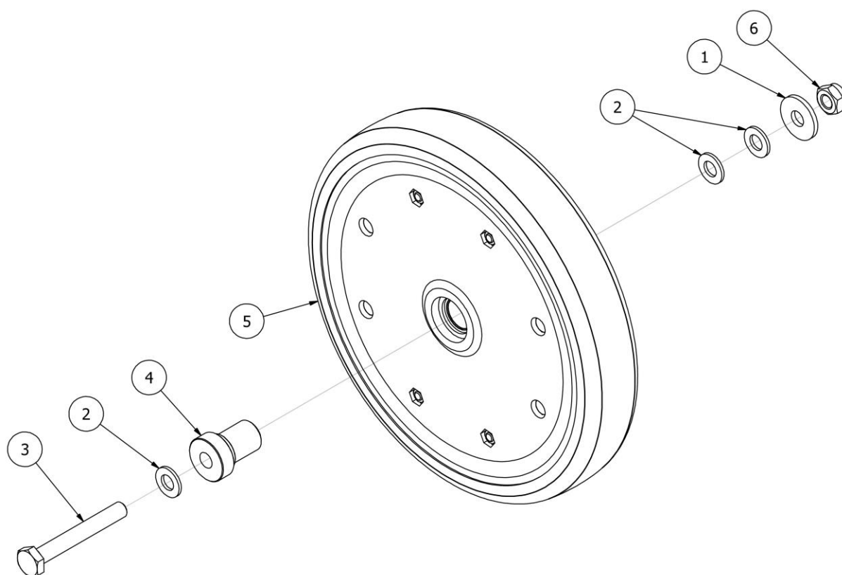
Rys. 1 SI00427 Koło kopiujące kompletne
