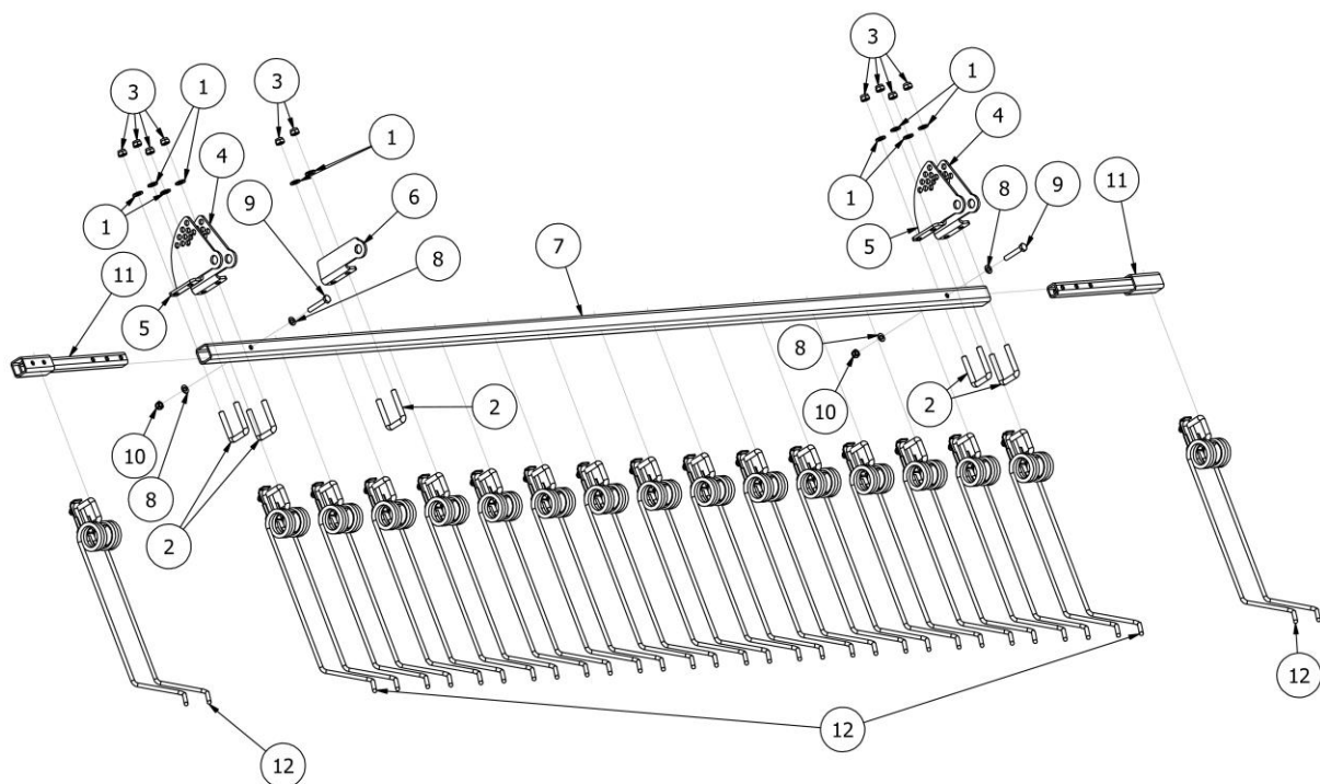
Rys. 15 SI02105 Zagarniacz z sprężynami SR300
