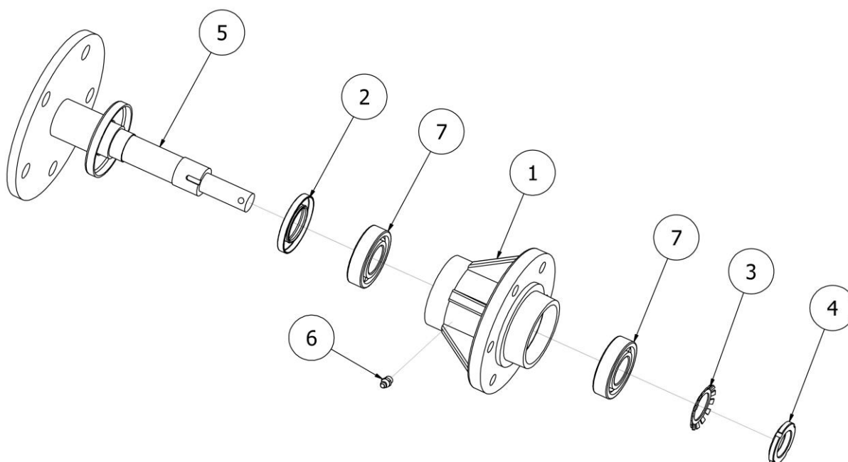
Rys. 5 SI04189 Piasta kompletna napędowa SR300 (prawa)
