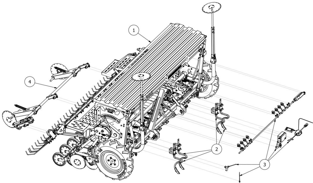
Rys. 1 SIM0041 – Siewnik rzędowy SR300
