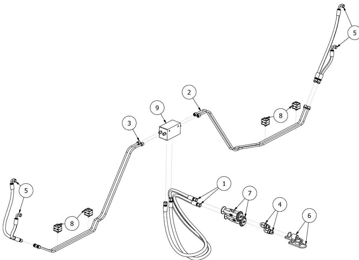
Rys. 10 HY00290 Układ hydrauliczny SR300
