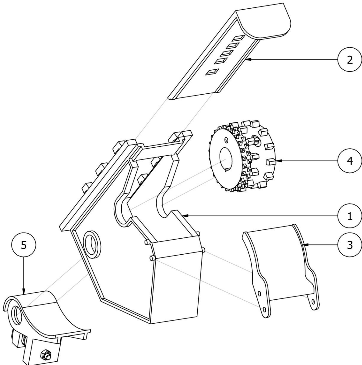
Rys. 11 SI00235 Aparat wysiewający kompletny
