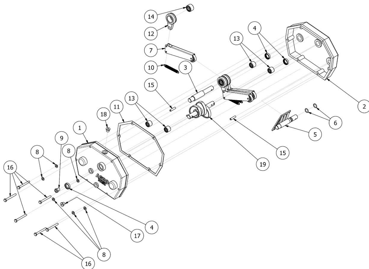
Rys. 13 SI00358 Skrzynia bezstopniowa
