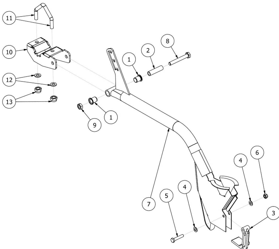
Rys. 38 SI01430 Redlica stopkowa prosta krótka kompletna (2016)
