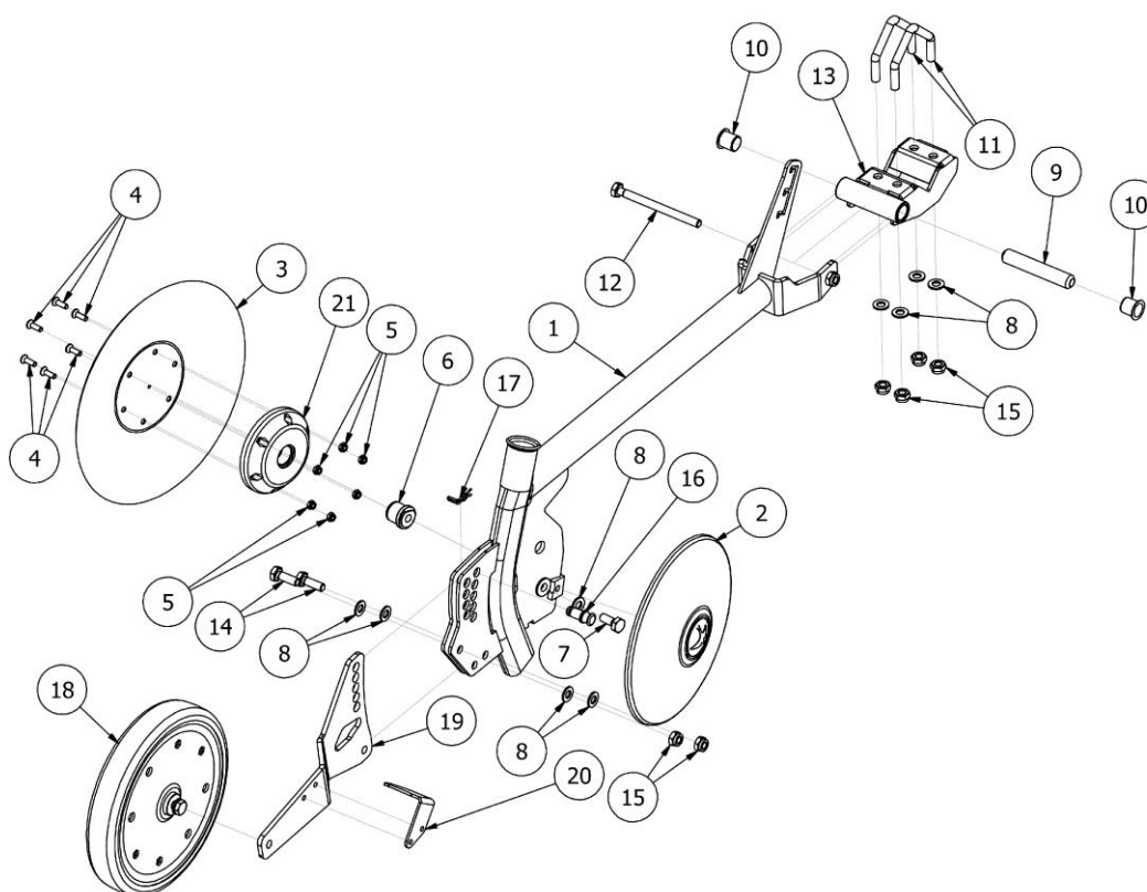
Rys. 32 SI01107 Redlica krótka prosta z talerzem czyszczącym kompletna
